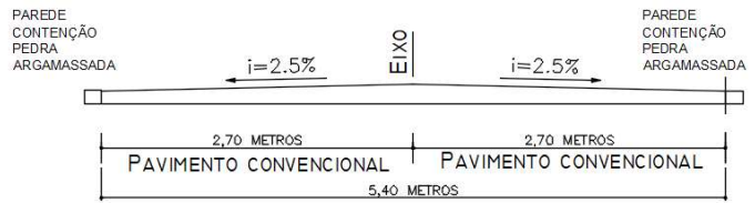
SEÇÃO TRANSVERSAL TIPO
