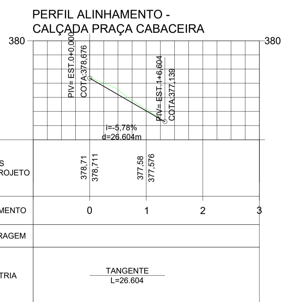
Perfil Longitudinal Escala Horizontal 1:800 Escala Vertical 1:100
