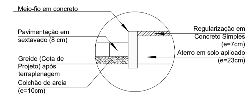
Detalhe 01 Escala 1:25
