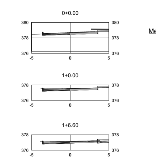
Perfis Transversais Escala 1:300
