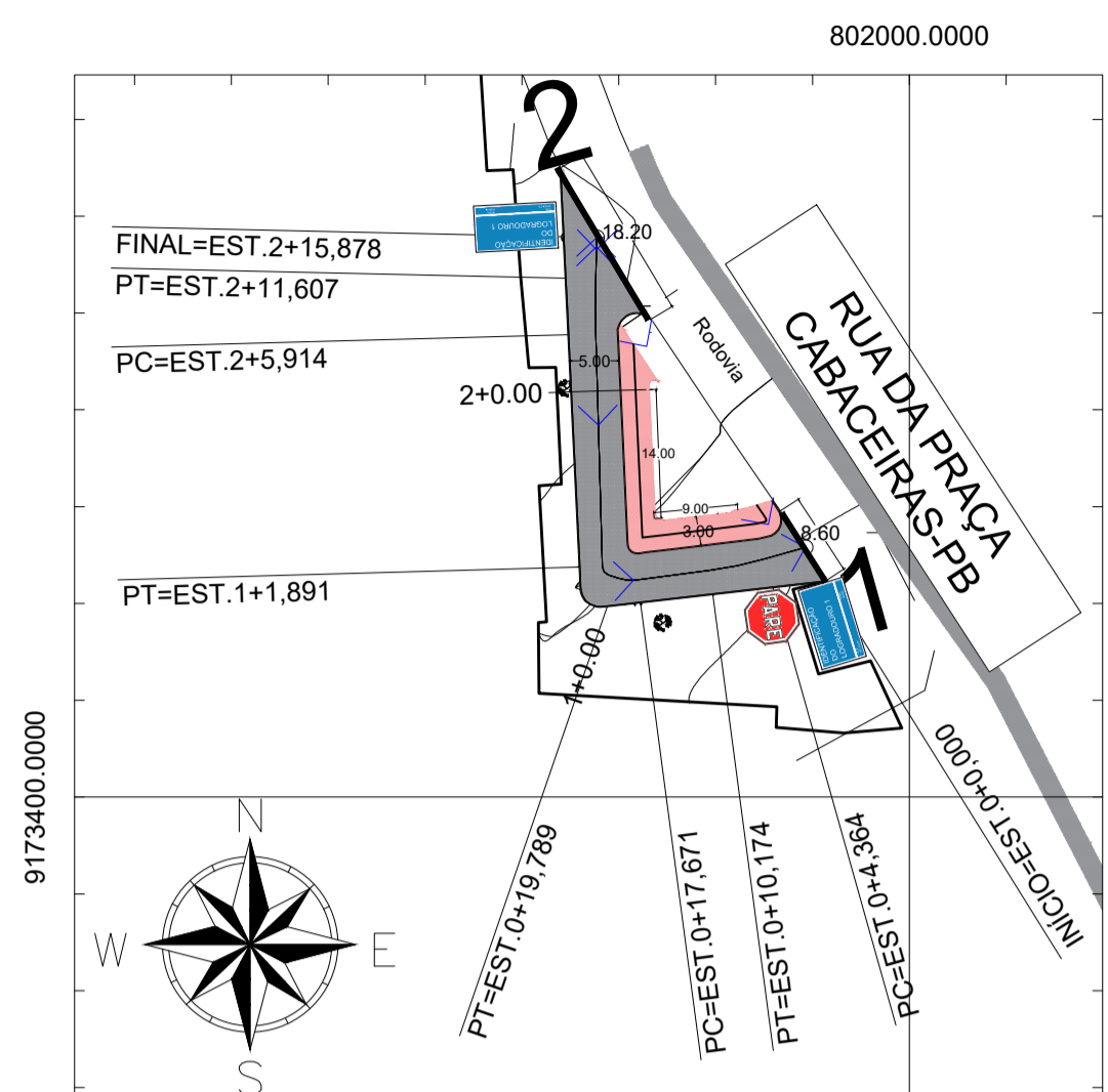
Planimetria Escala 1:800
