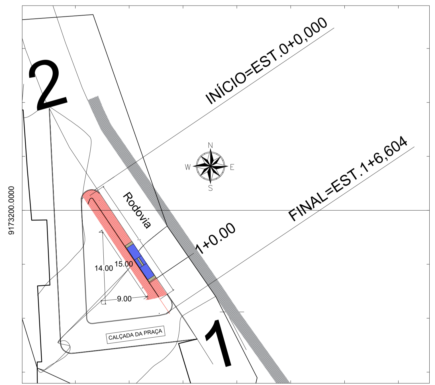
Planimetria - Praça Escala 1:400
