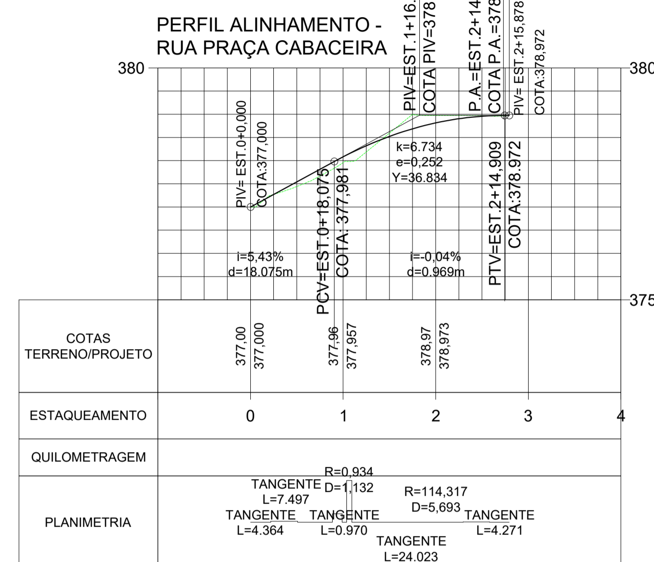
Perfil Longitudinal Escala Horizontal 1:800 Escala Vertical 1:100
