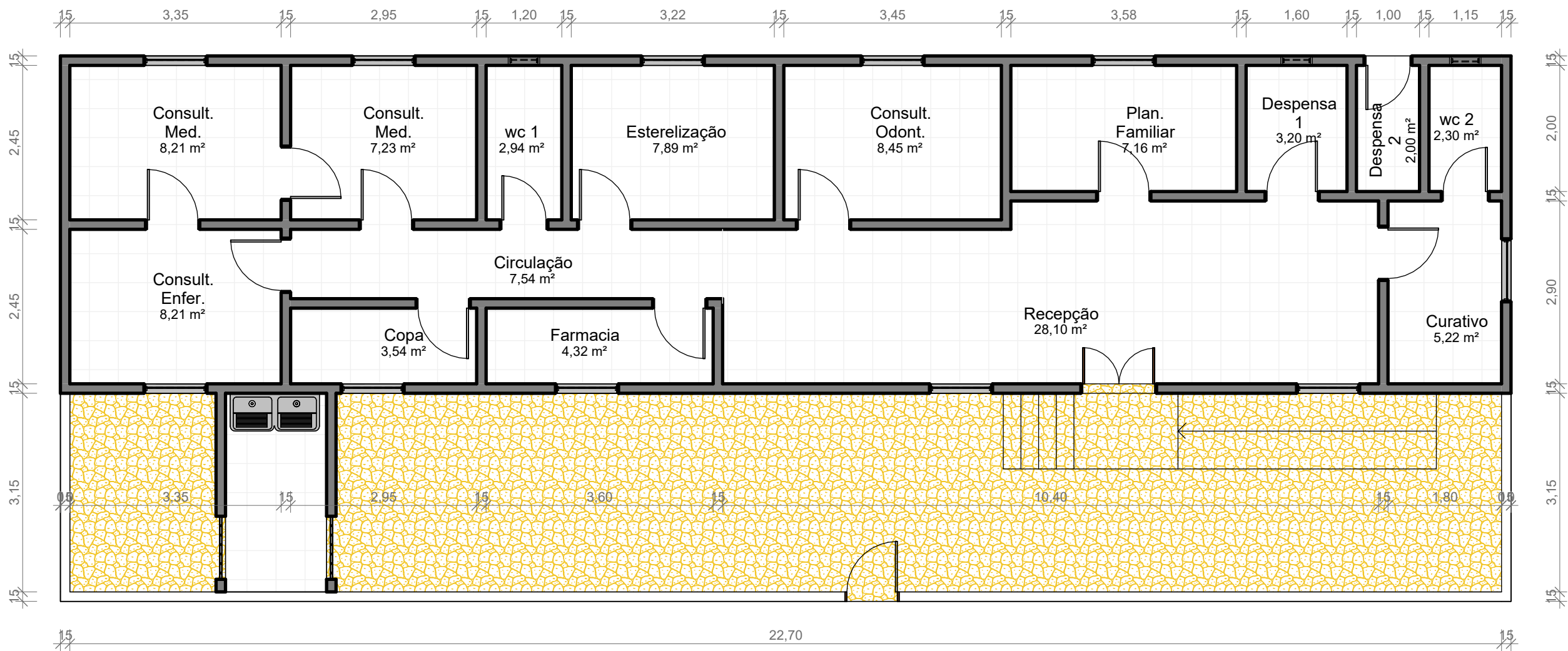
1 PLANTA BAIXA TÉRREO ESCALA 1 : 75
