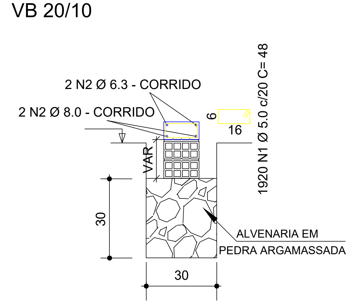
5 DETALHAMENTO EMBASAMENTO MURO Escala: 1/50
