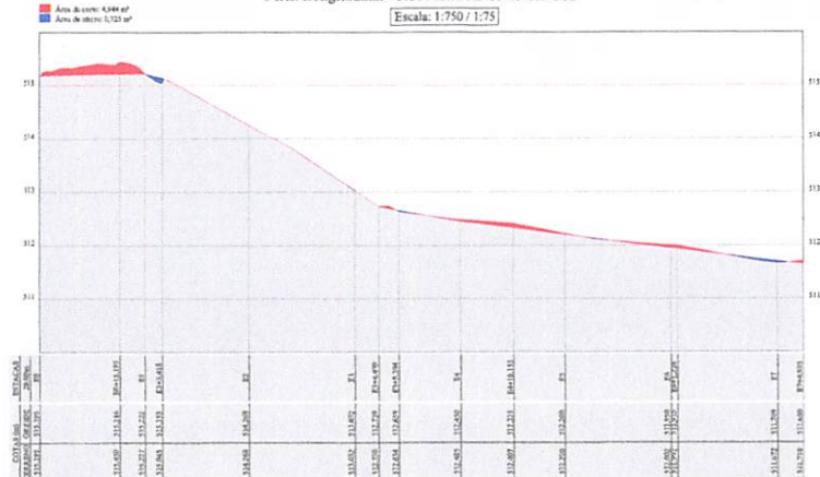
Perfil Longitudinal - Rua Maria Alves de Oliveira
