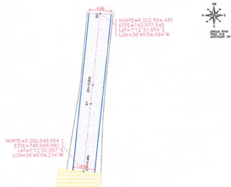
PLANALTIMETRIA Escala: 1:500
