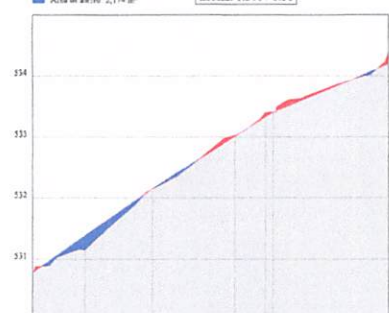
Perfil Longitudinal - Trav. Martinho Cardoso Andrade Área de corte: 1,592 m 2 Área de aterro: 2,174 m 2 Escala: 1:500 / 1:50
