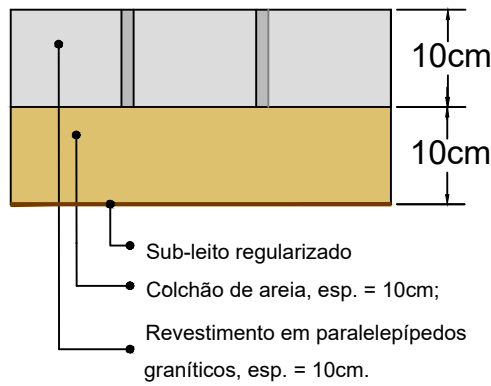
MÉTODO CONSTRUTIVO - PAVIMENTAÇÃO DAS RUAS - PARALELEPÍPEDO SEM ESCALA
