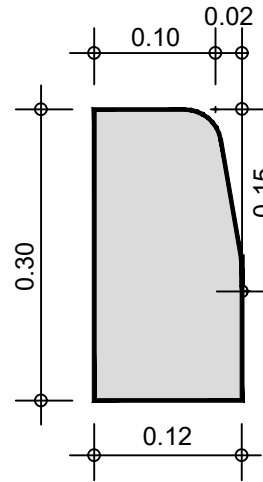
MEIO-FIO PRÉ-MOLDADO S/ESCALA
