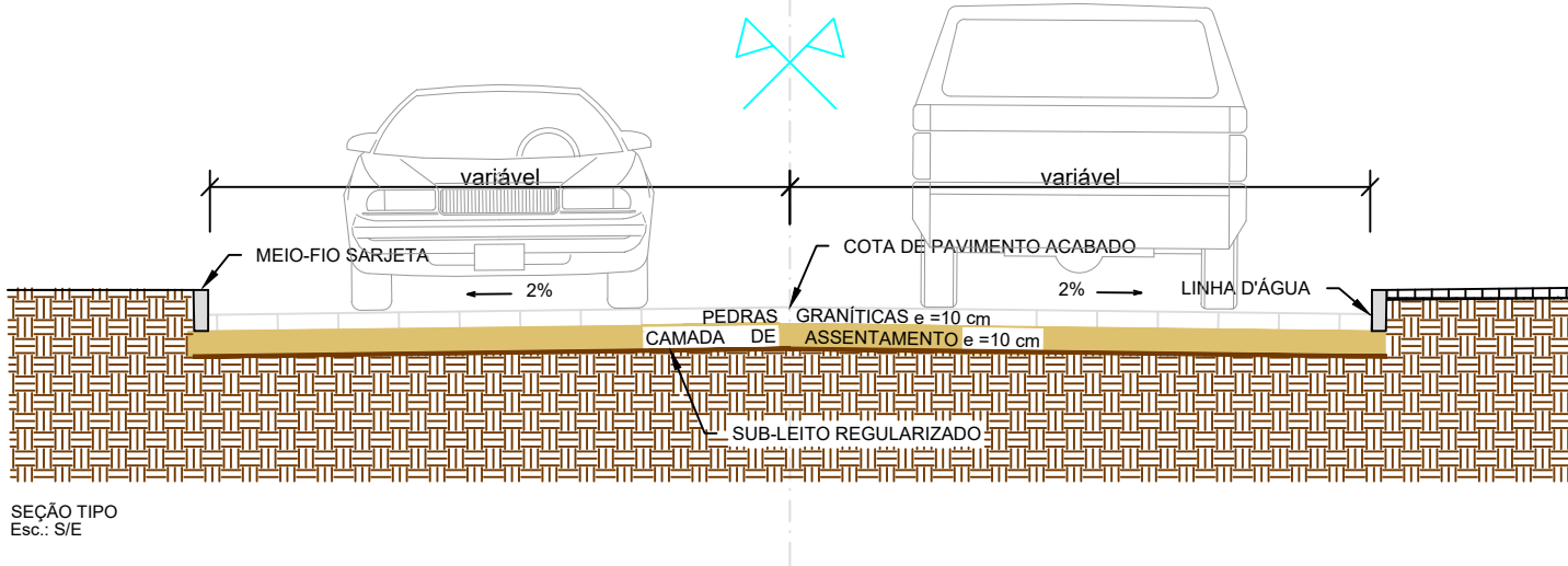
PAVIMENTAÇÃO EM PARALELEPÍPEDO
