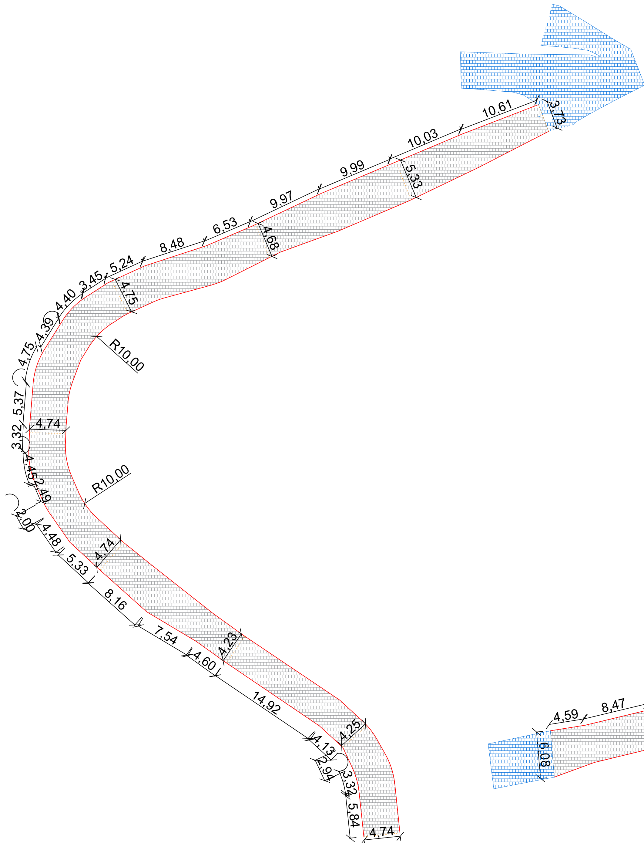
TRECHO 17 (153,00m) Área 728m² PLANTA BAIXA PAVIMENTAÇÃO ESC 1:300
