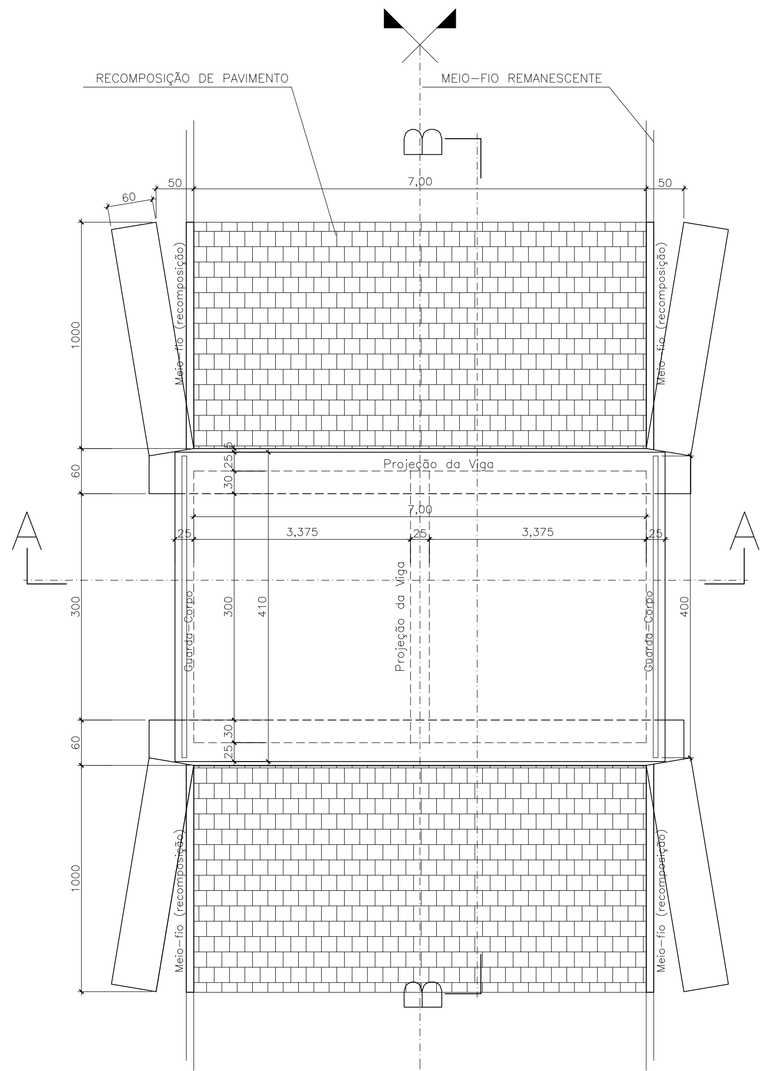
PLANTA BAIXA — VISTA SUPERIOR ESCALA: 1/50
