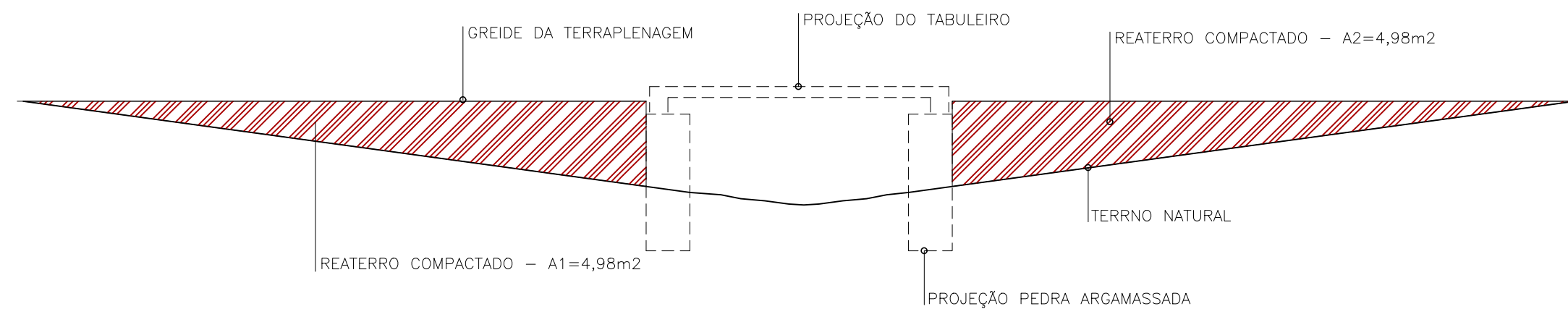
SEÇÃO LONGITUDINAL — ATERRO ESCALA: 1/75
