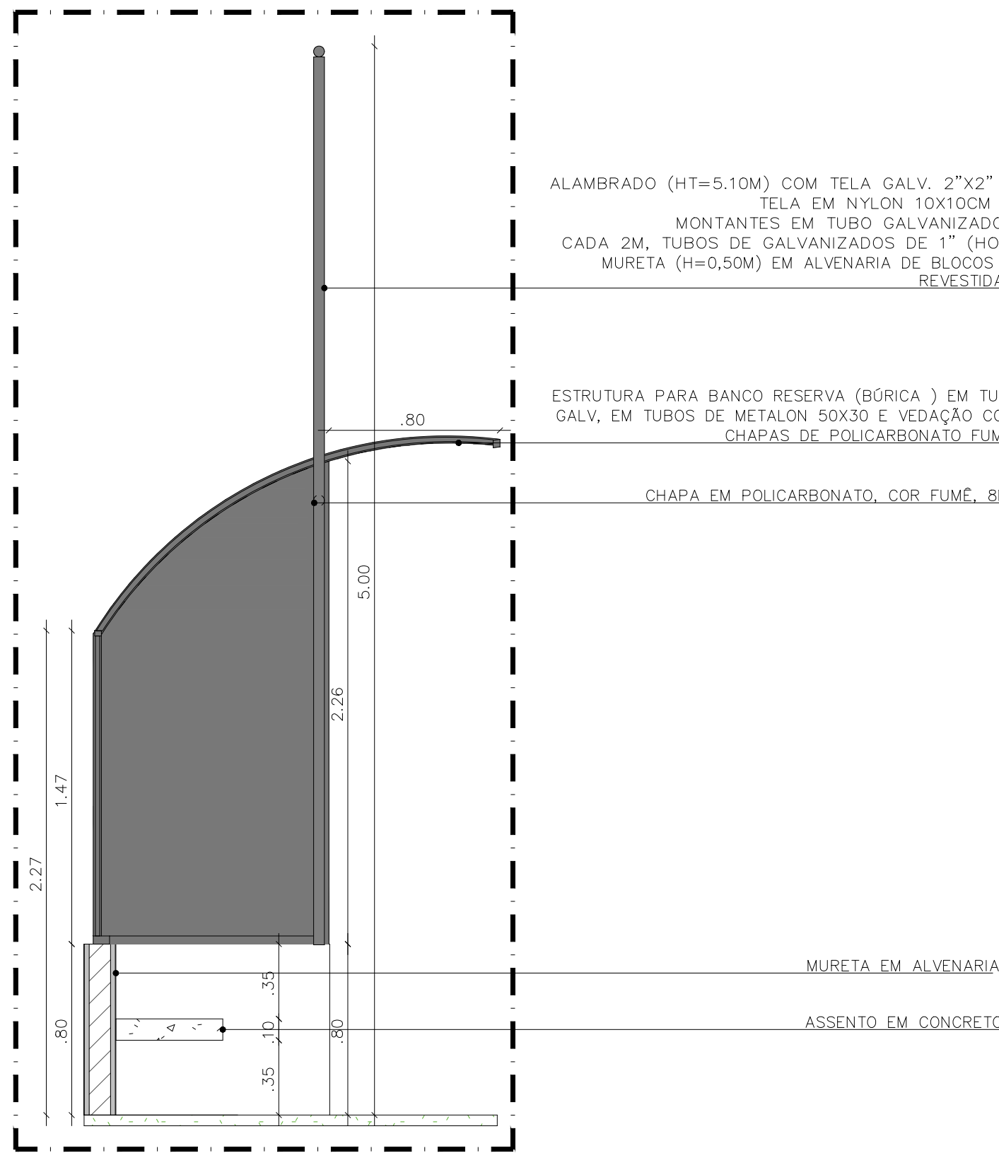
CORTE AA'
