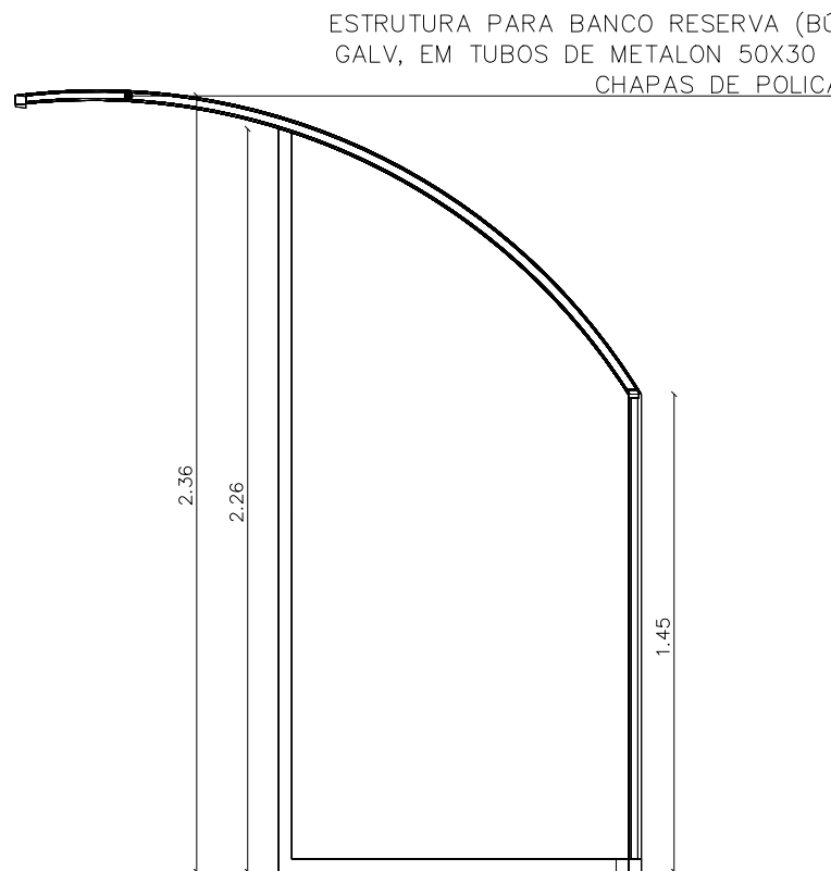
CORTE BB'
