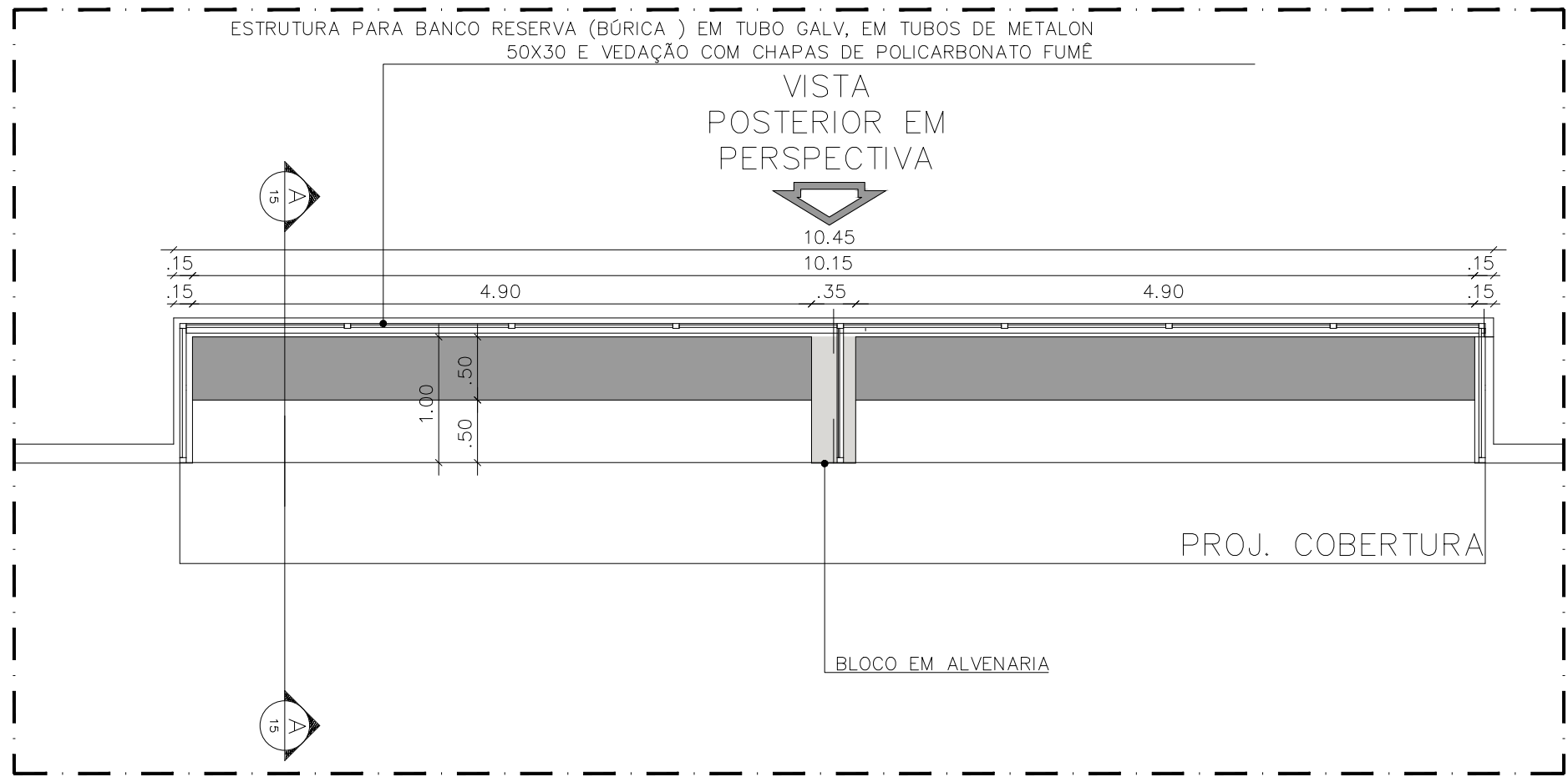
PLANTA BAIXA - COBERTURA DO BANCO DE RESERVA
