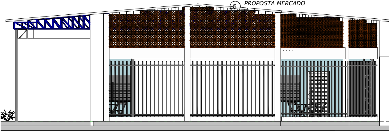
3 FACHADA OESTE 1 : 50
