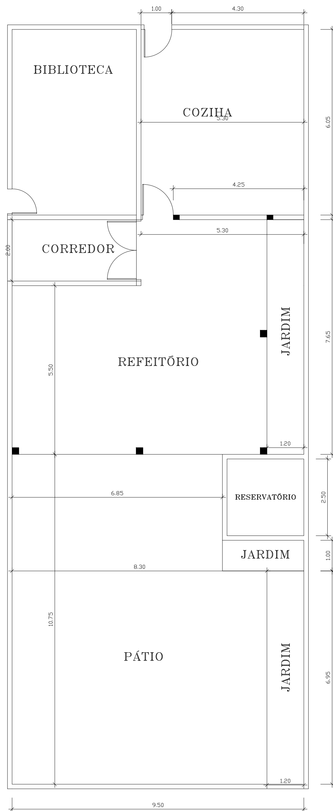
PLANTA BAIXA ESCALA 1:50
