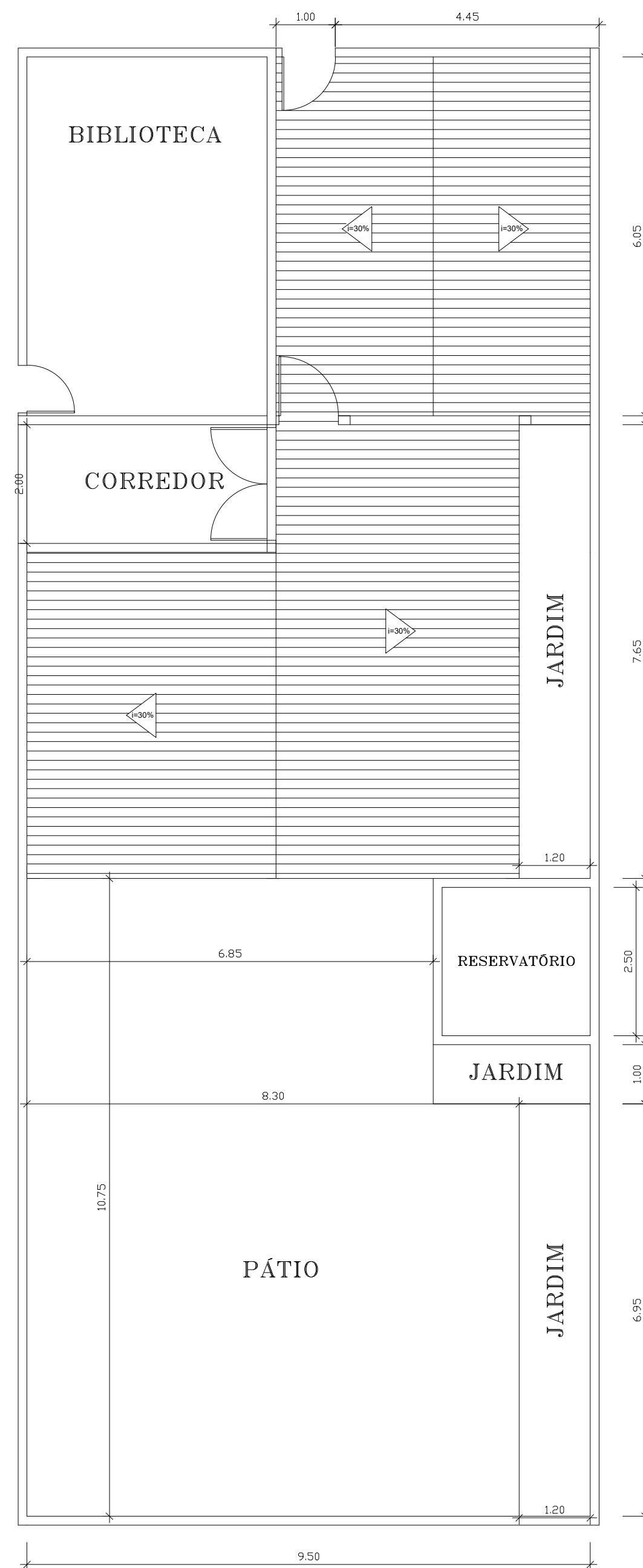
PLANTA DE COBERTA ESCALA 1:50
