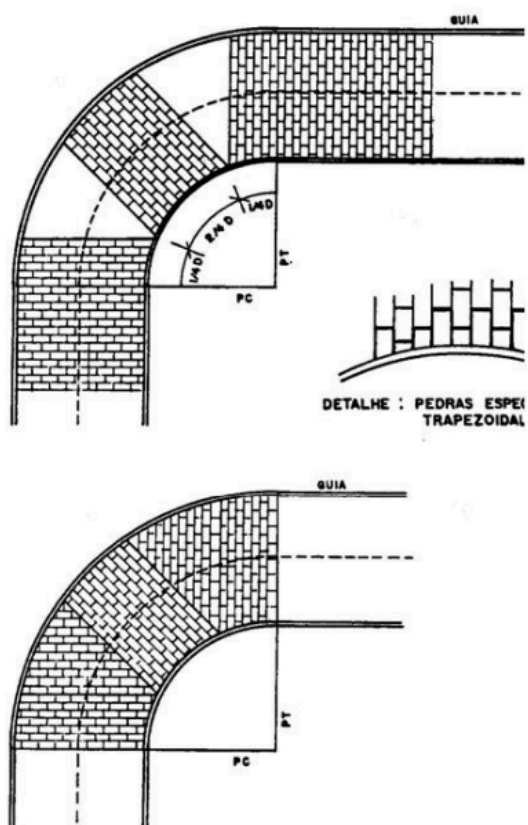
Figura 03. Trecho em Curva de Pequeno Raio
