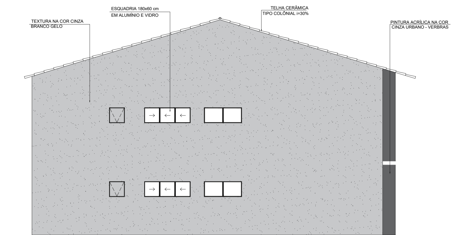
2 FACHADA 03 ESCALA 1/75
