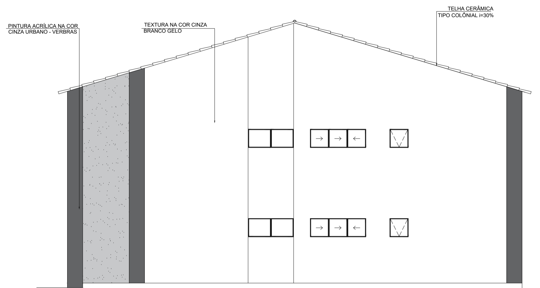
1 FACHADA 02 ESCALA 1/75
