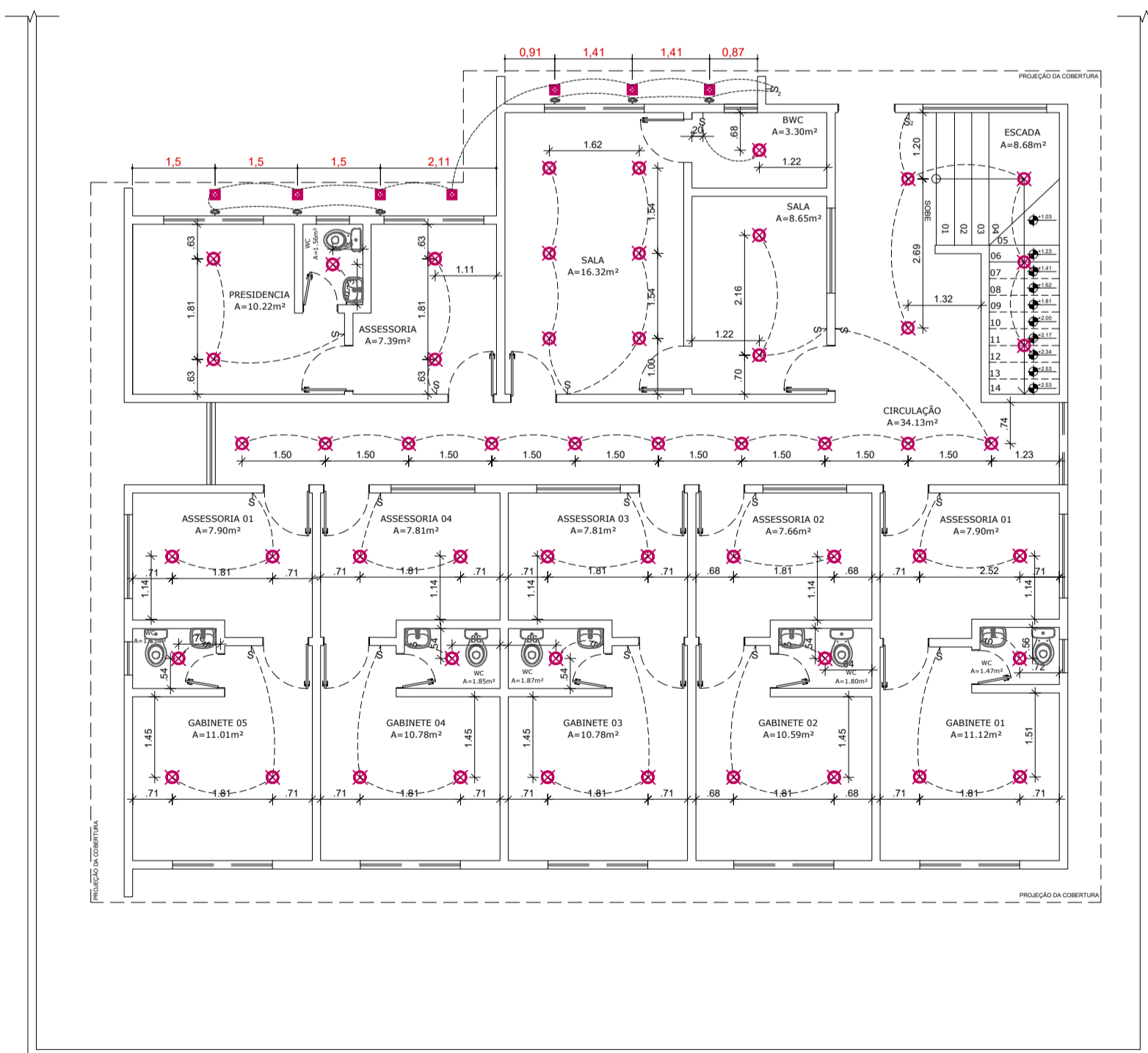
3 PLANTA BAIXA ELÉTRICA - TÉRREO ESCALA 1/100
