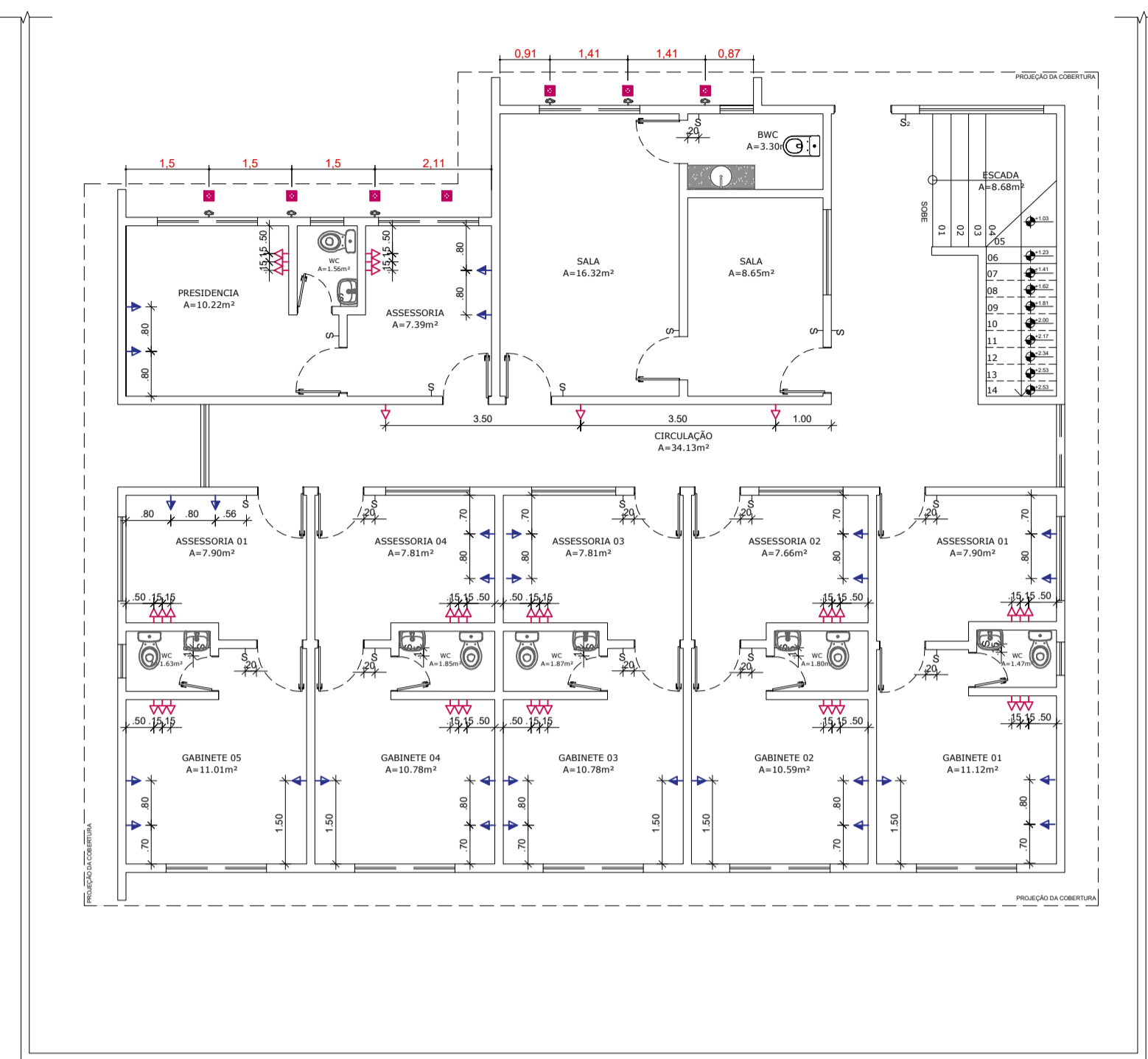
1 PLANTA BAIXA ELÉTRICA - TÉRREO ESCALA 1/100
