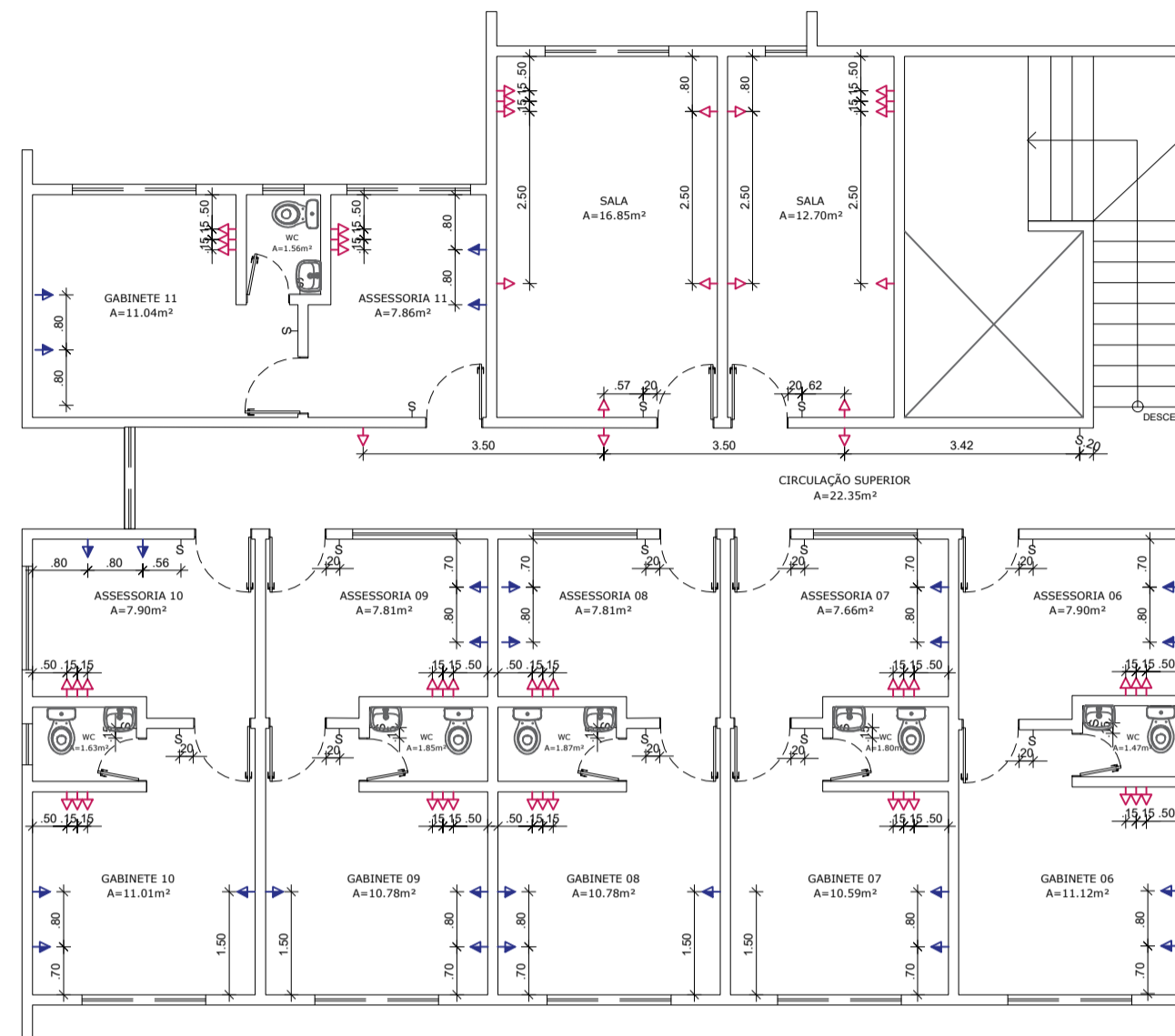
2 PLANTA BAIXA ELÉTRICA - PAV. SUPERIOR ESCALA 1/100
