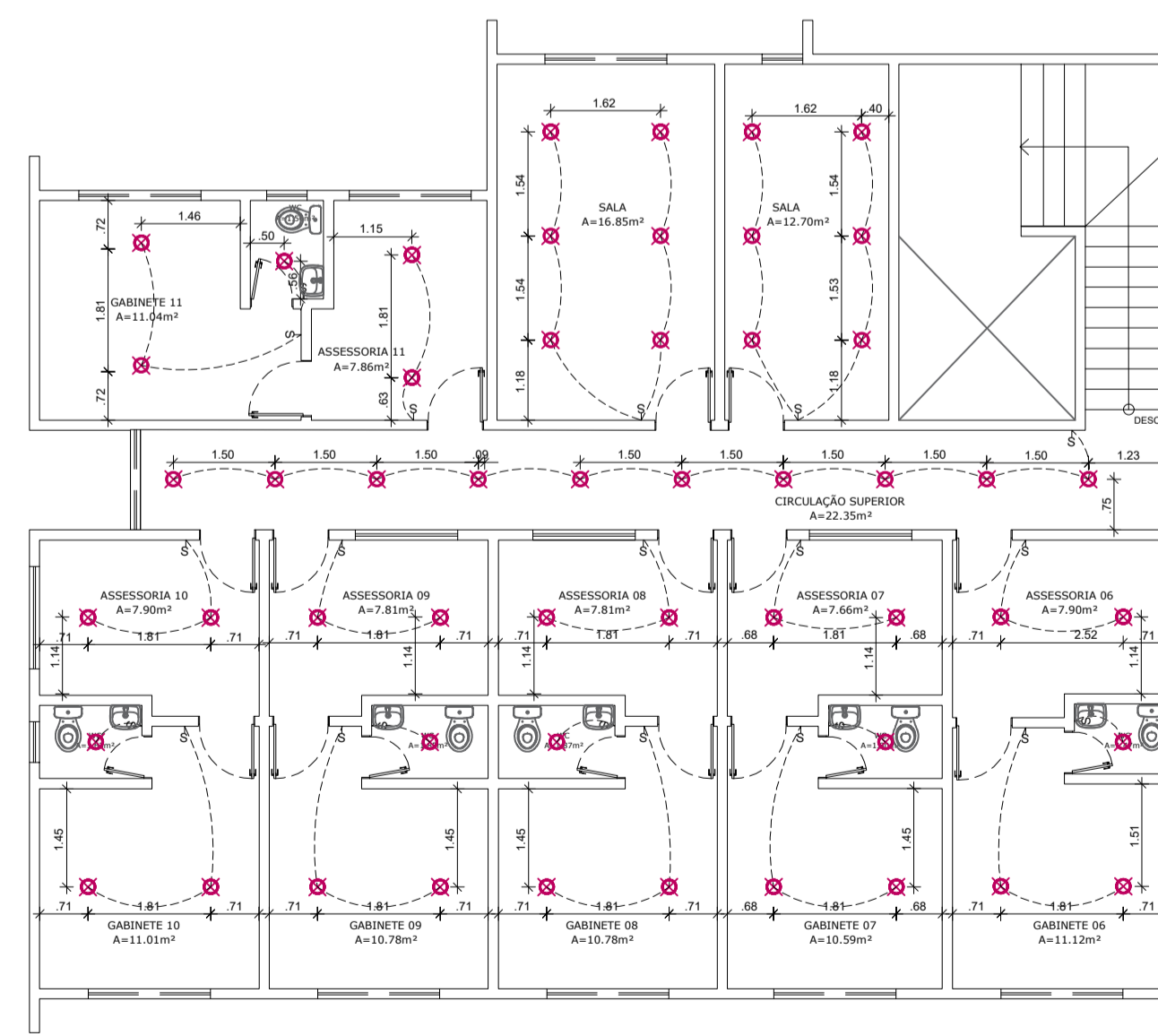
4 PLANTA BAIXA ELÉTRICA - PAV. SUPERIOR ESCALA 1/100
