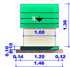
3 CORTE B CACHORRO 1 : 25
