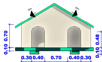
2 CORTE A CACHORRO 1 : 25
