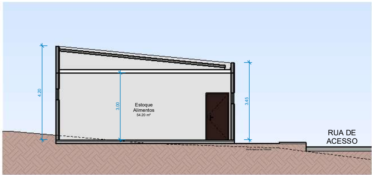
04 CORTE AA ESCALA 1:75
