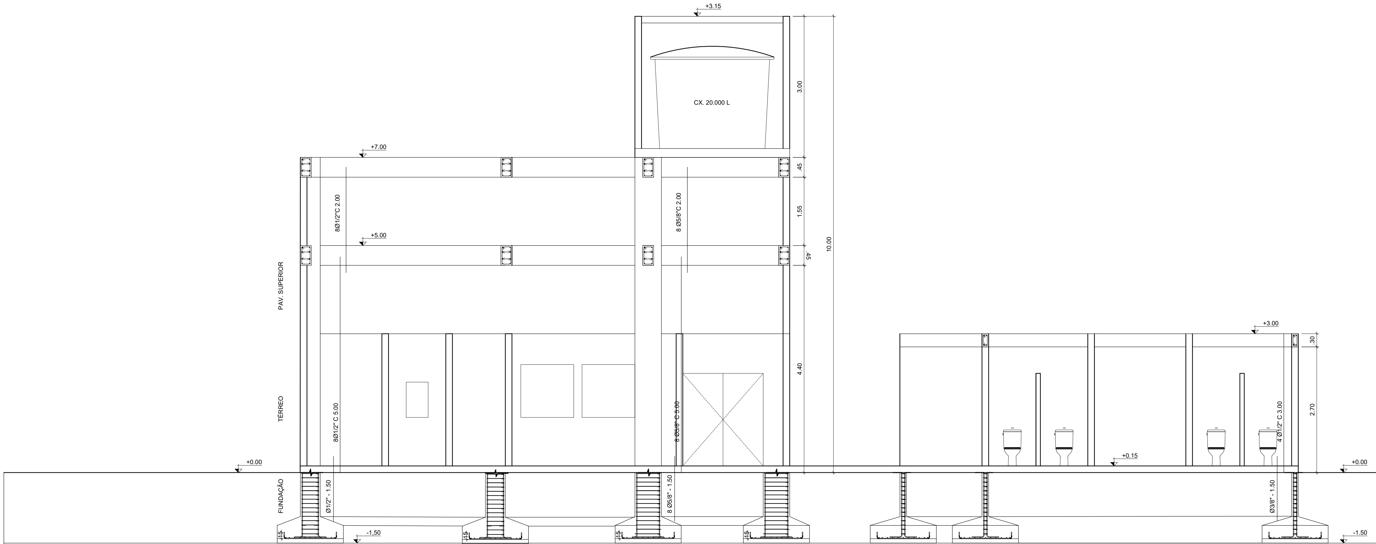
CORTE AA' MATADOURO PÚBLICO ESTRUTURA escala 1/50
