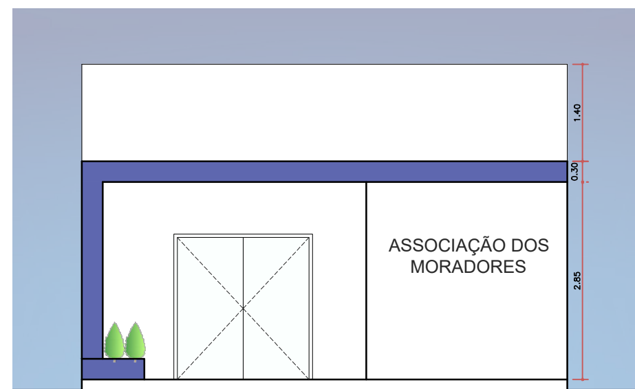
FACHADA FRONTAL ESC. 1:50
