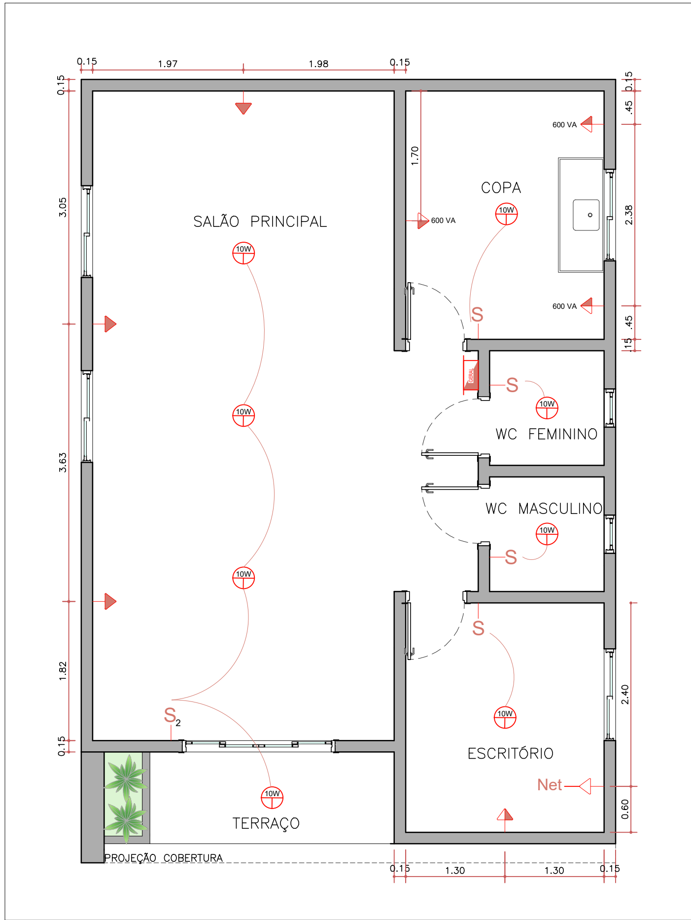
PLANTA BAIXA TÉRREO ESC. 1:50
