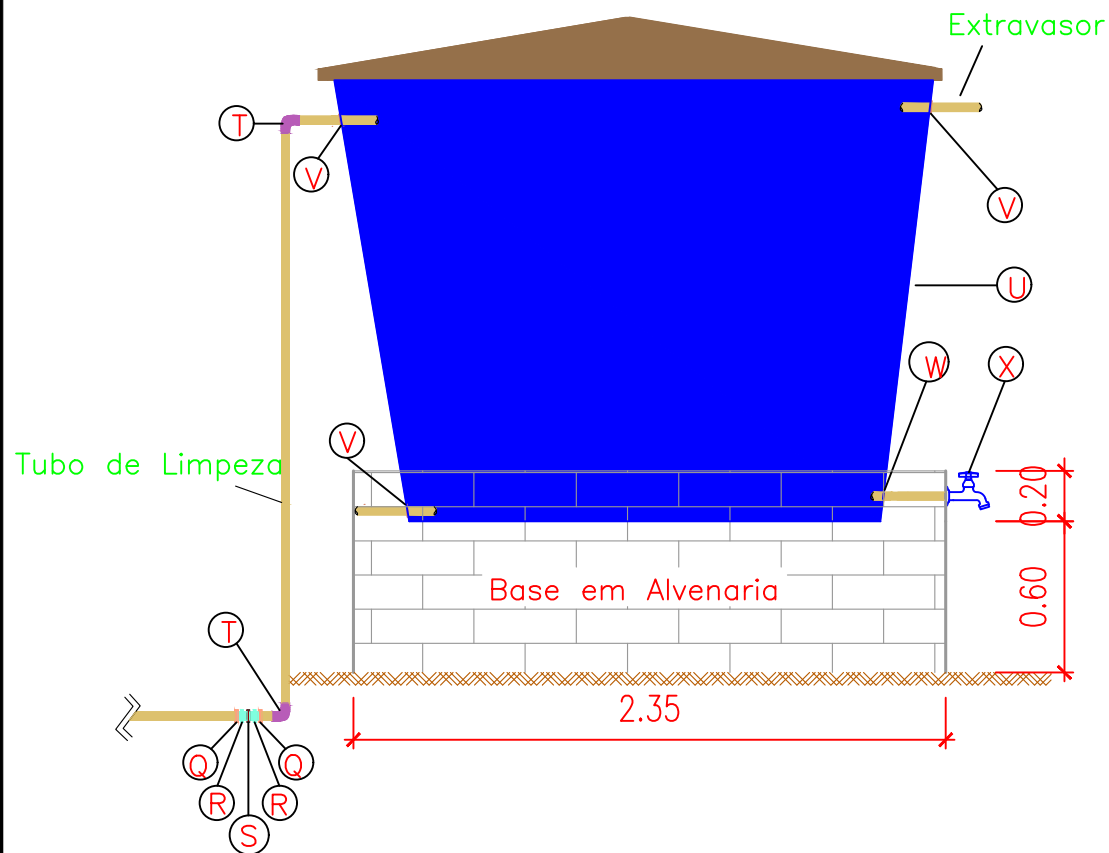
DETALHE DA CAIXA ESC 1:30
