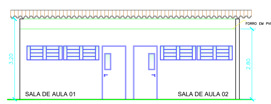
01 VISTA A ESCALA 1/100
