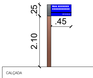
PLACA DE IDENTIFICAÇÃO DA RUA ESC _____ 1/25
