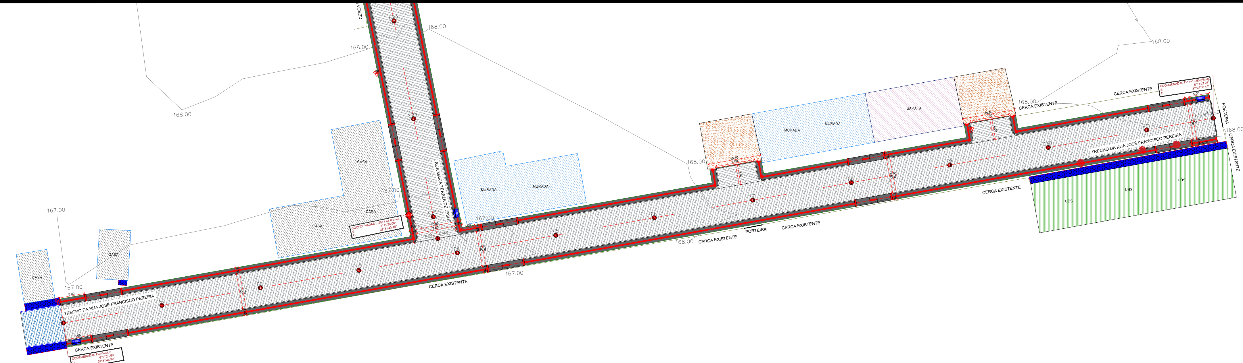
PLANTA DE SITUAÇÃO - RUA JOSÉ FRANCISCO PEREIRA DETALHE 01 - TRECHO 02 ESCALA 1/300
