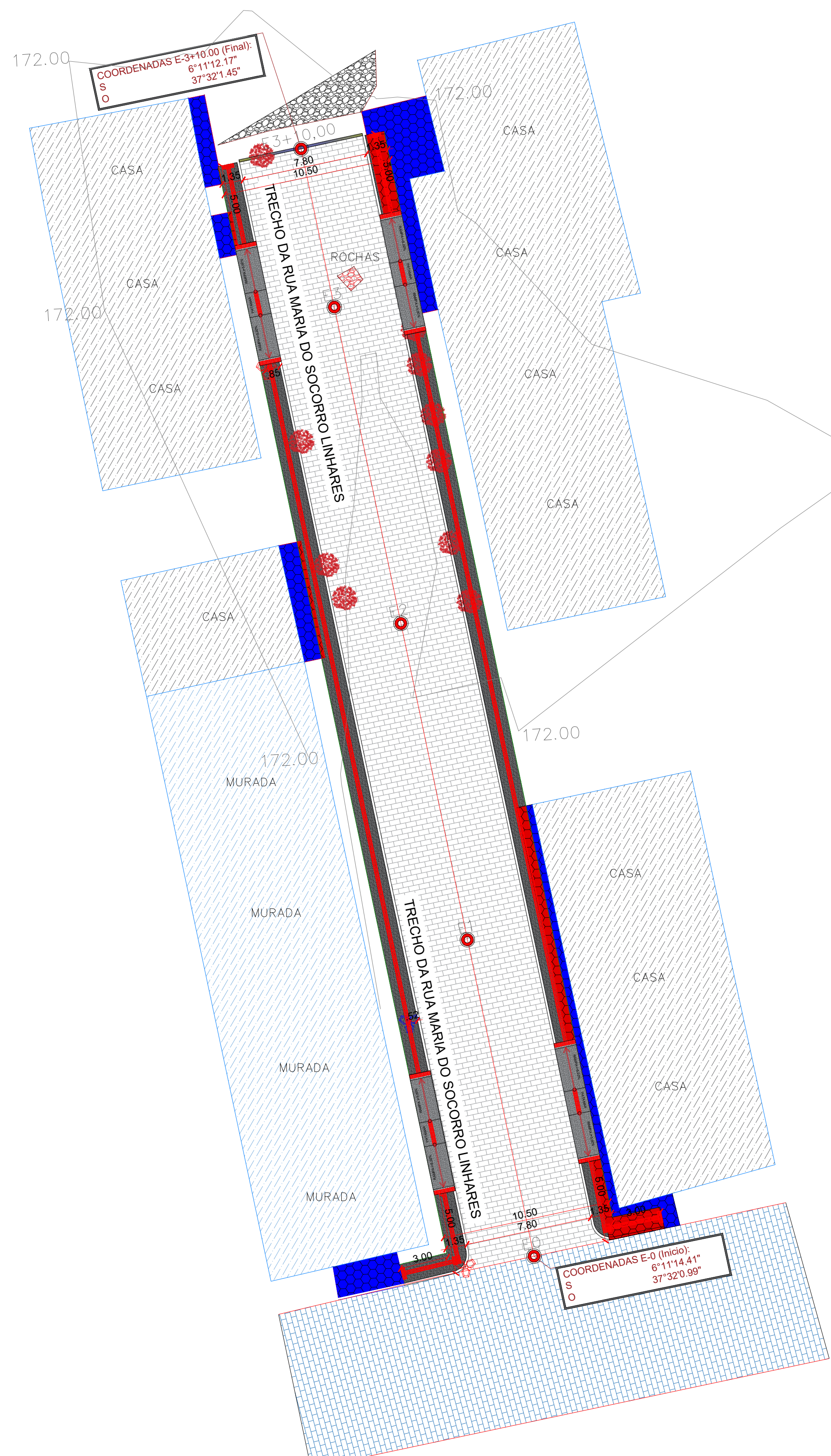
PLANTA DE SITUAÇÃO - GERAL ESCALA 1/200
