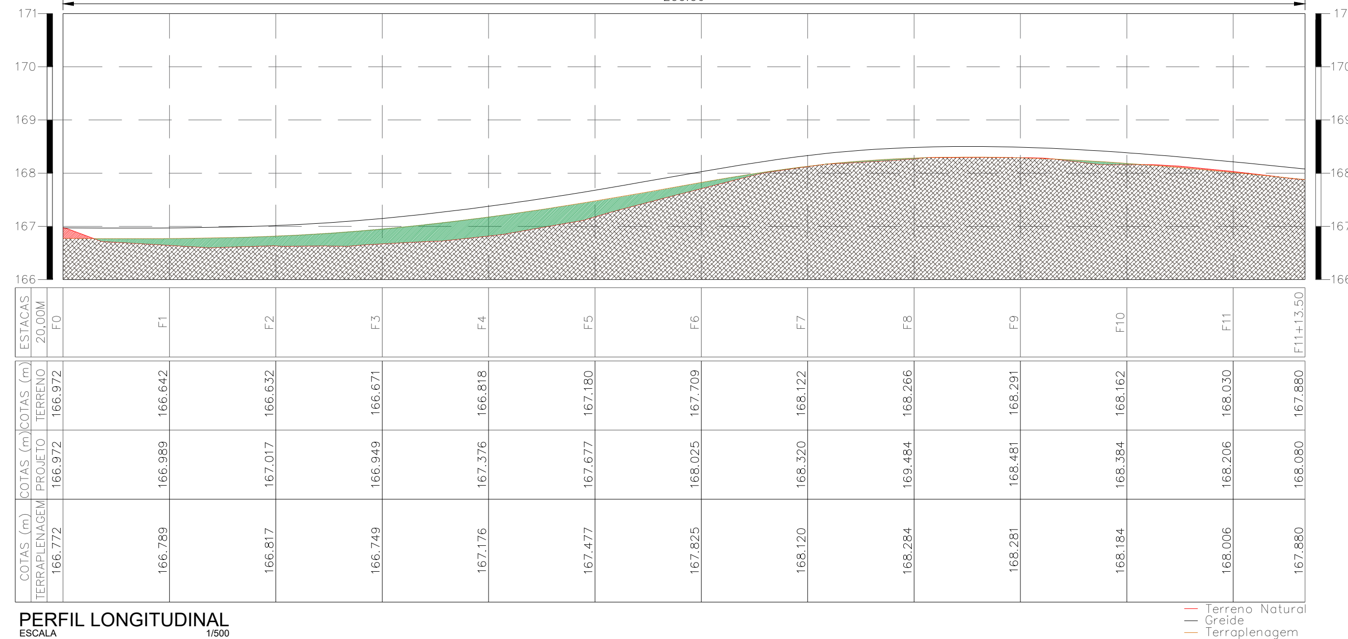
Trecho da Rua José Francisco Pereira Perfil Longitudinal Escala: H.....1/5.000 V.....1/500 233.50
