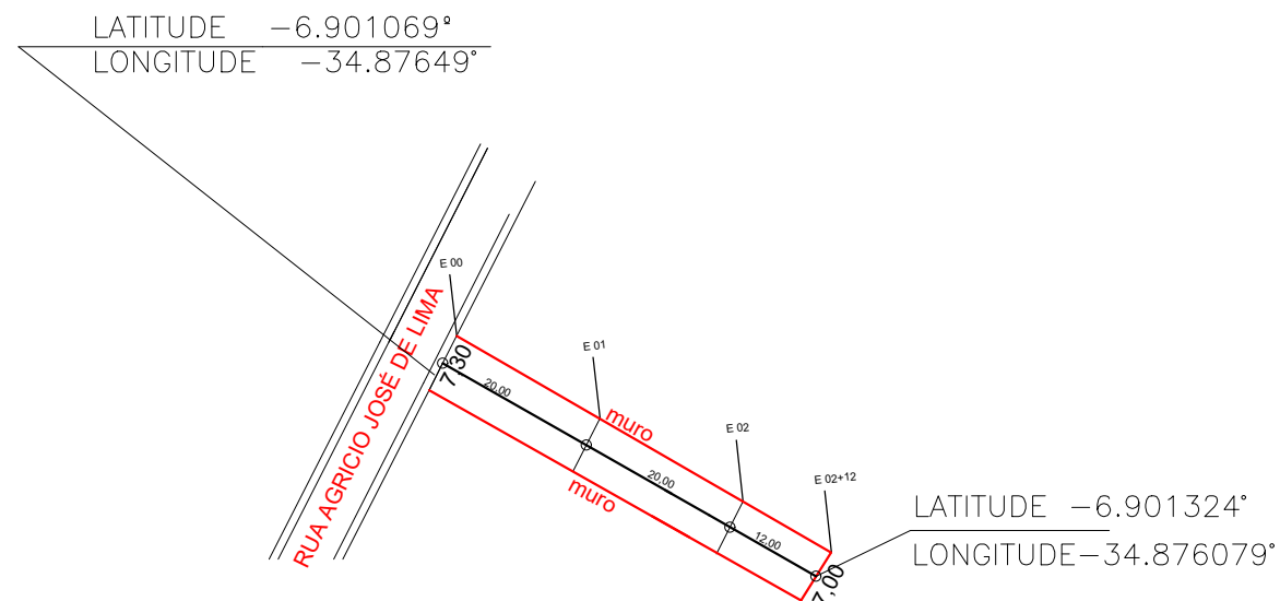
CAMINHAMENTO ESCALA --1/1000
