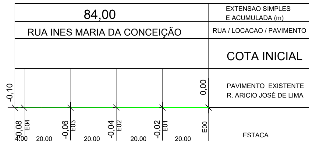
PERFIL - LONGITUDINAL ESCALA --1/1000
