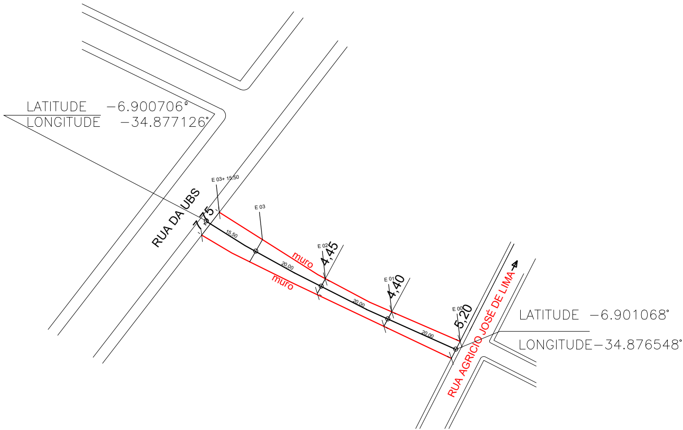
CAMINHAMENTO ESCALA --1/1000
