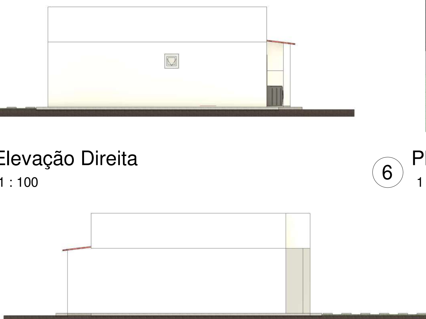
9 Elevação Esquerda 1 : 100
