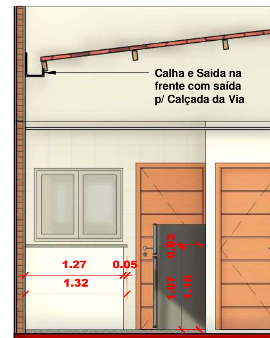
13 DET - Balcão Americano 1 : 50
