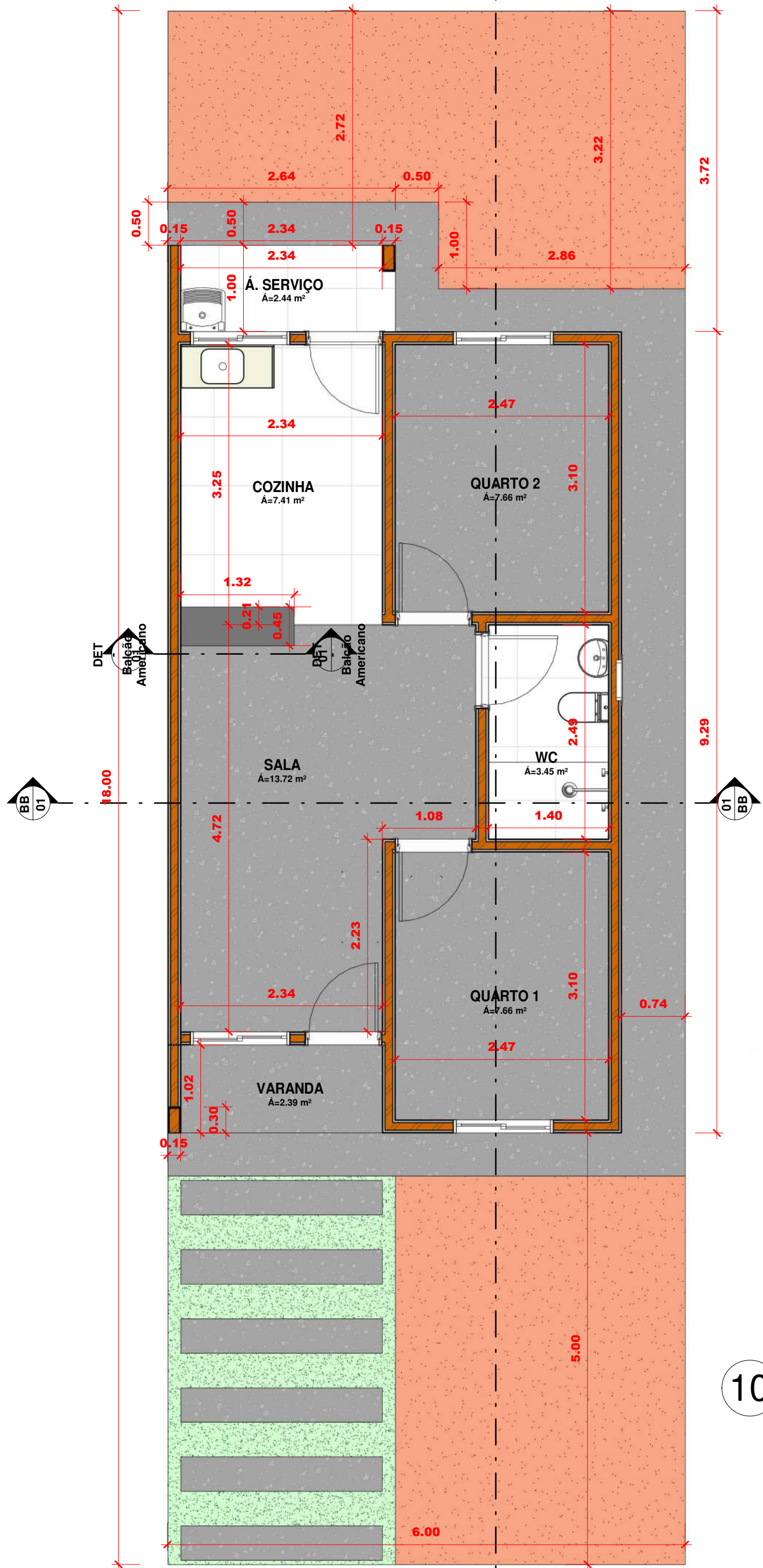
1 Planta Baixa - Térreo 1 : 50
