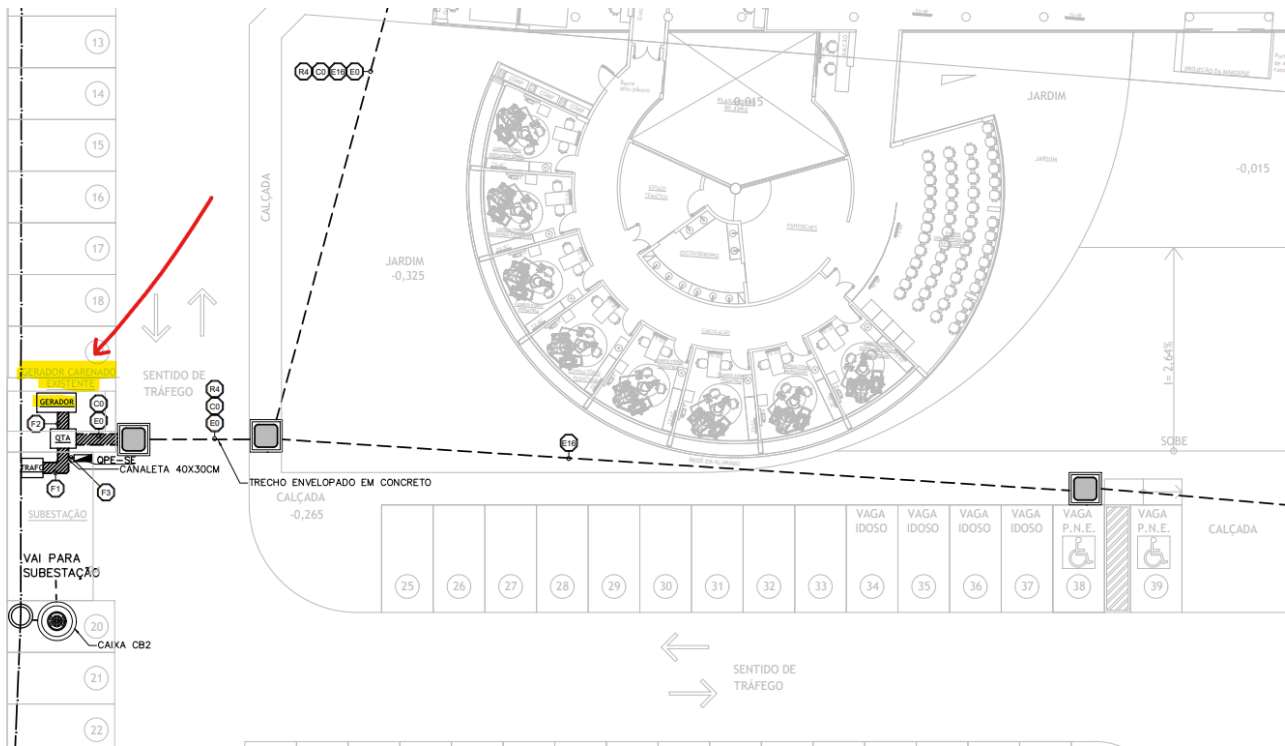
Figura 1. Trecho da PLANTA Nº 01/32 - PROJETO EXECUTIVO - SUBESTAÇÃO & GERADOR (Doc. SEI 117852579).
