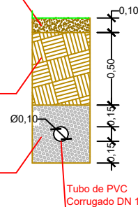
DETALHE DE INSTALAÇÃO DOS DRENOS SEM ESCALA
