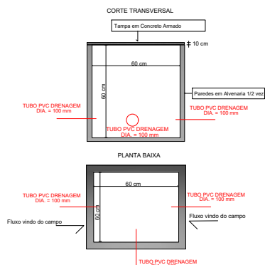
DETALHE CAIXA DE PASSAGEM SEM ESCALA
