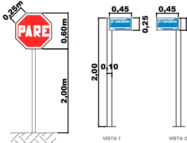
Detalhe de Placa de Sinalização
