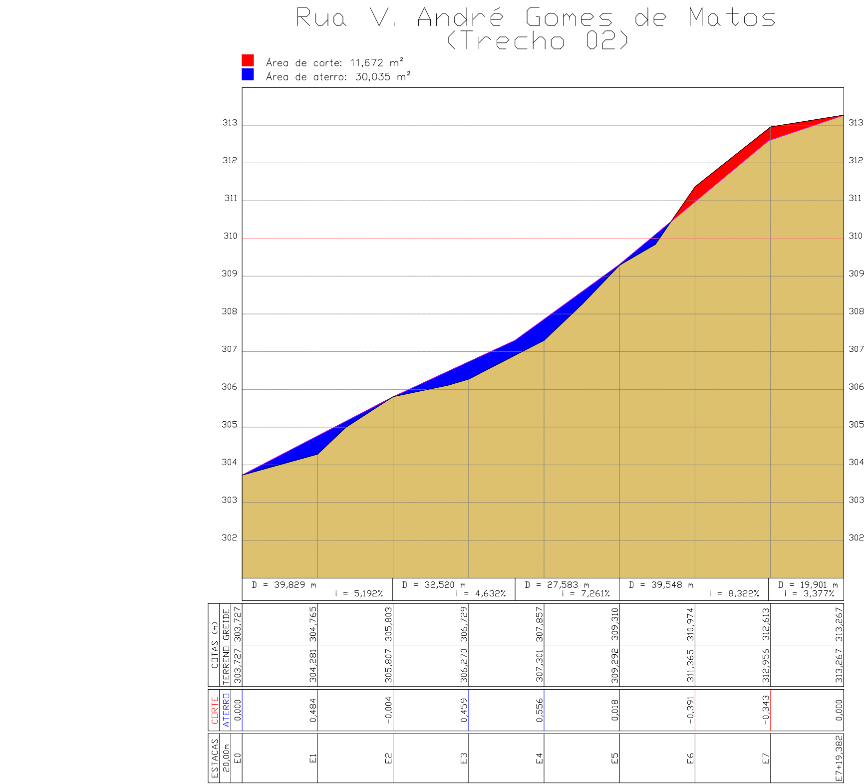
PERFIL LONGITUDINAL Esc. 1:1000
