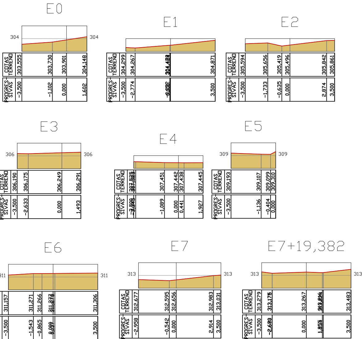
SEÇÃO TRANSVERSAL
