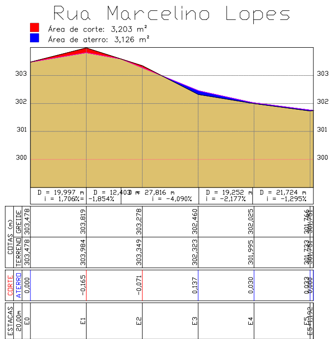
PERFIL LONGITUDINAL Esc. 1:1250
