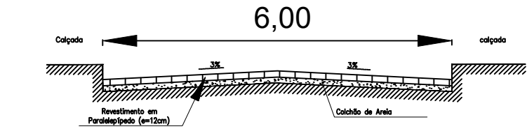
SEÇÃO TRANSVERSAL TIPO
