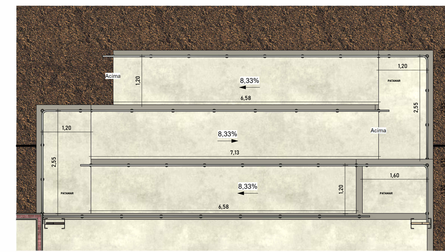
4 CO - TÉRREO 1:50
