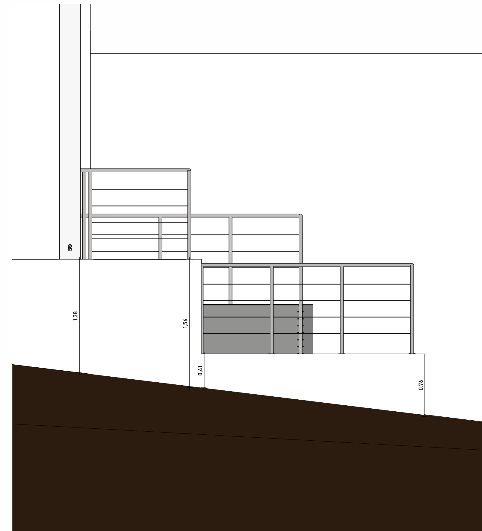
3 CO - LESTE 1:25
