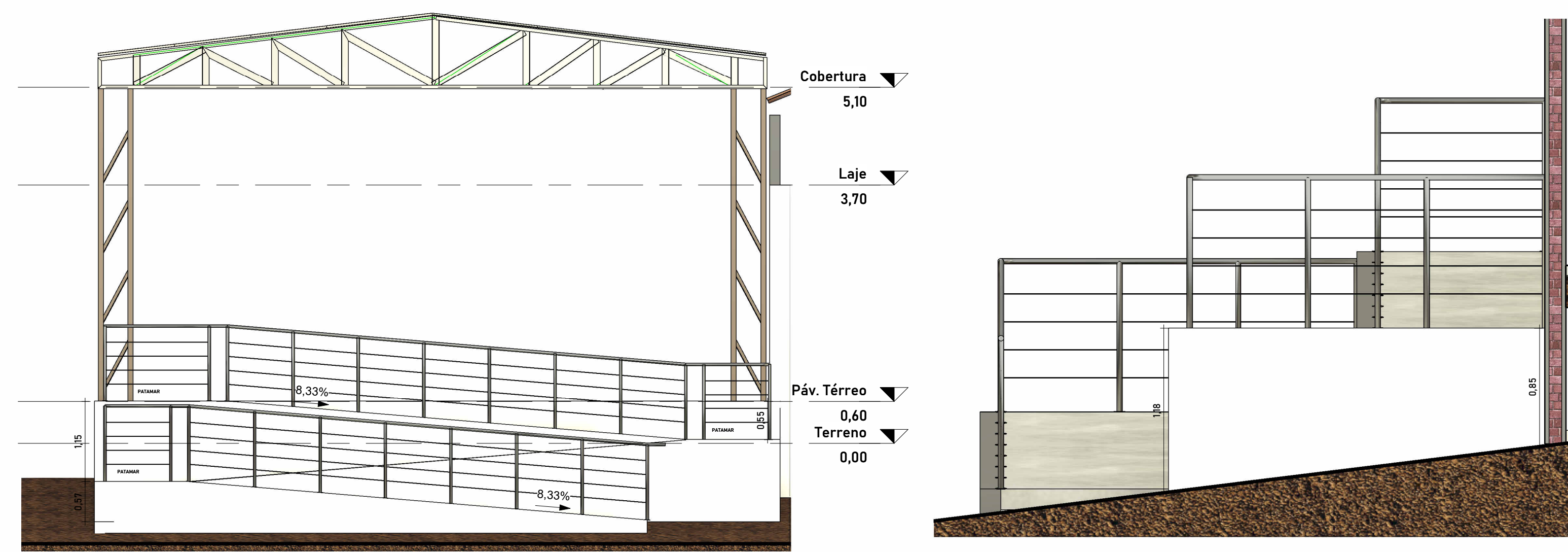
1 Corte 1 1:50
