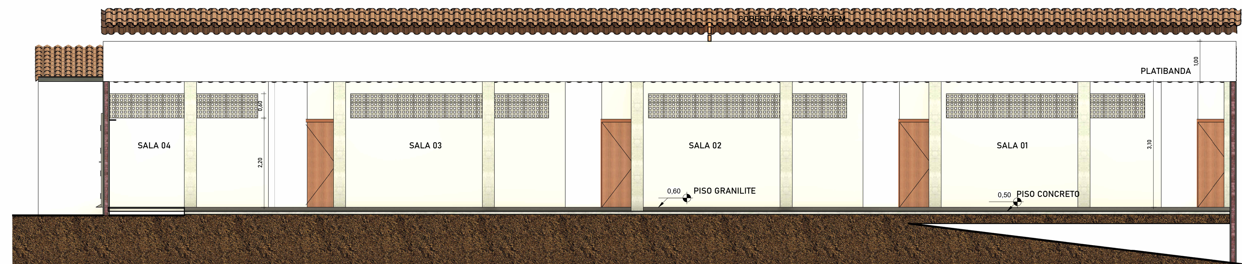
7 Corte 4 1:50
