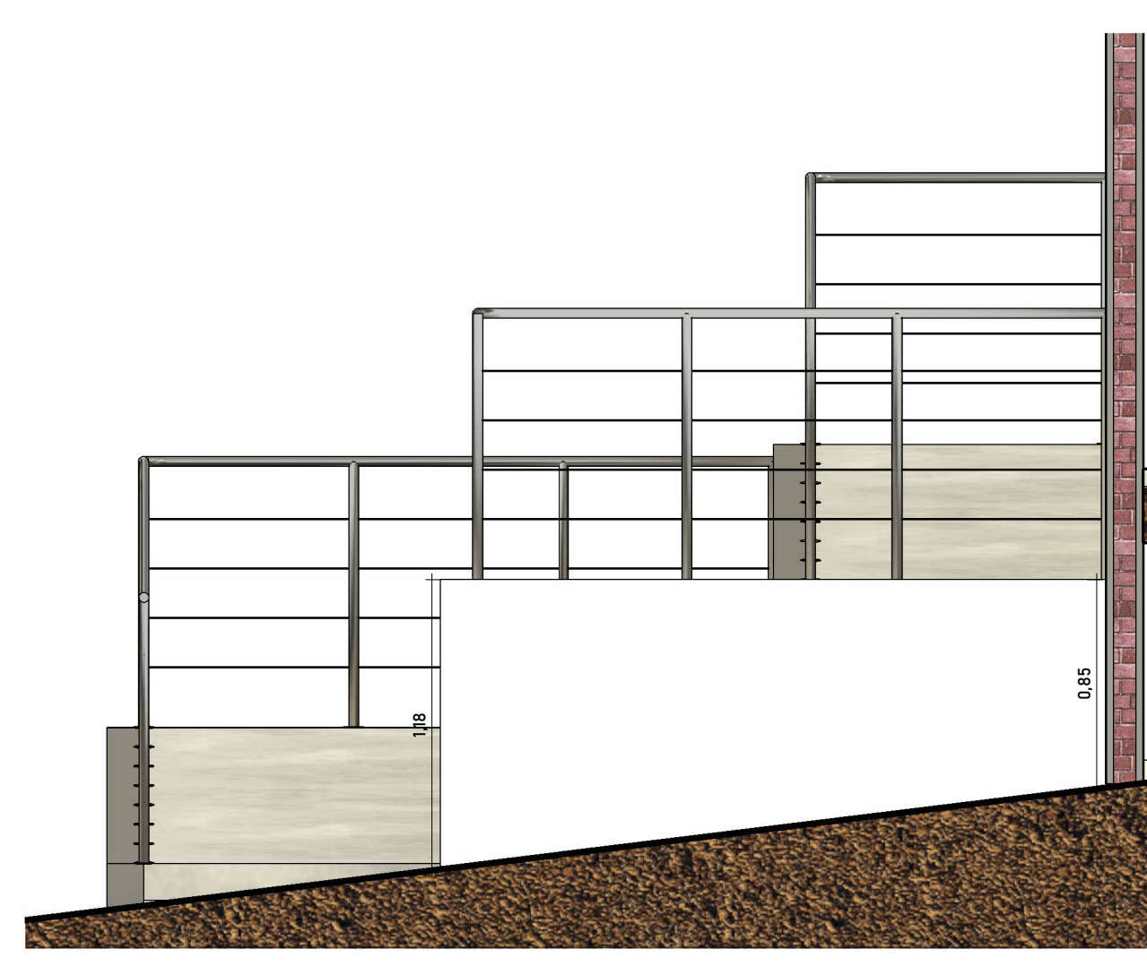
2 Corte 2 1:25
