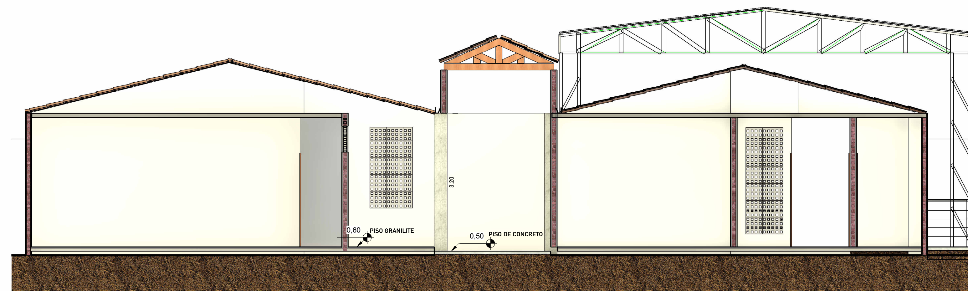
6 Corte 3 1:50
