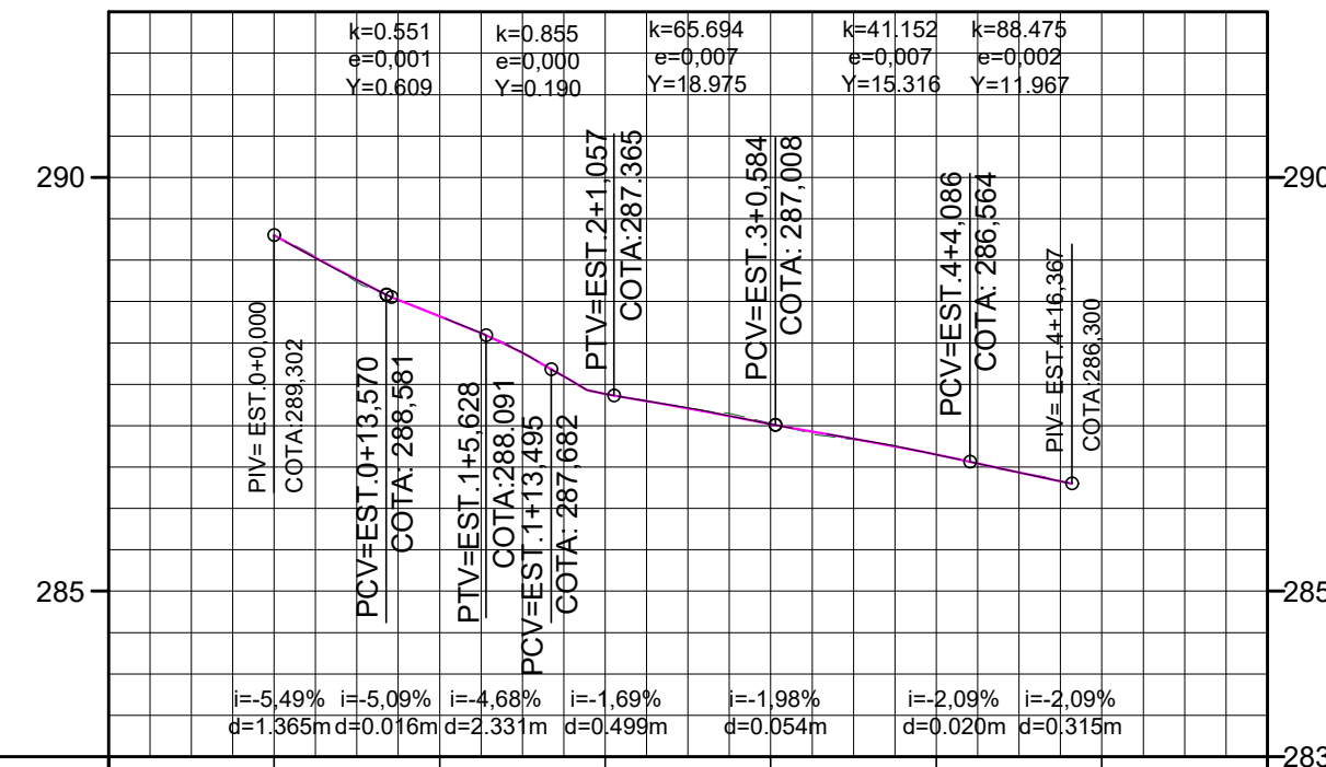
PERFIL ALINHAMENTO - RUA PROJETADA 28
