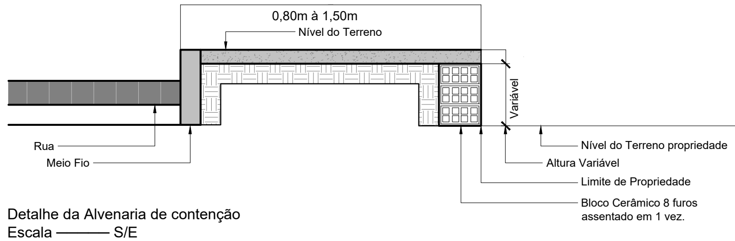
Detalhe da Alvenaria de contenção Escala — S/E
