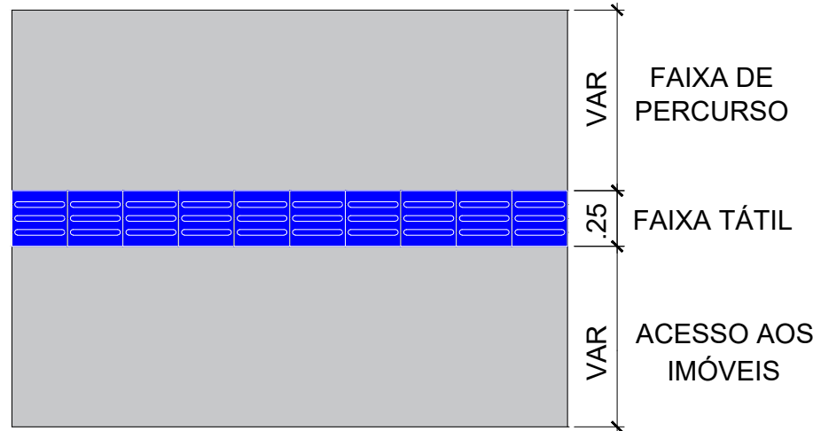
Detalhe do Piso Tátil Escala — S/E
