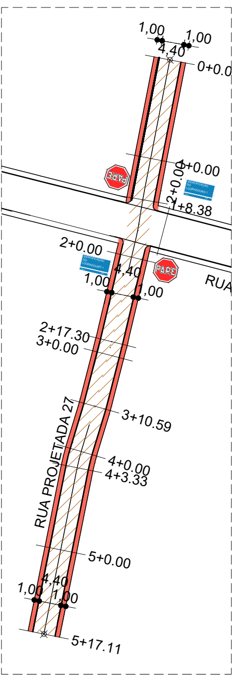
Planimetria Escala 1:750
