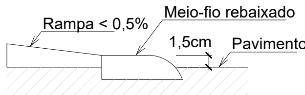
Detalhe Meio fio Escala — S/E
