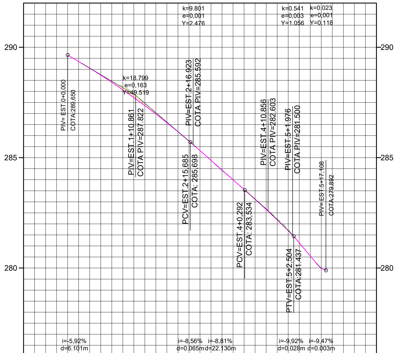
PERFIL ALINHAMENTO - RUA PROJETADA 27
