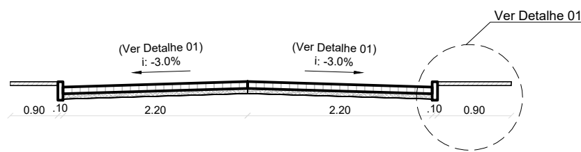
Seção Transversal Tipo Escala 1:100
