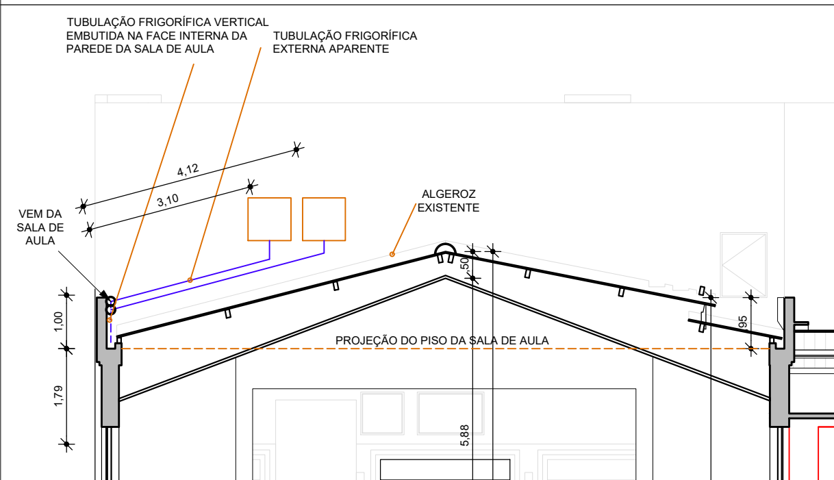
CORTE A.A
