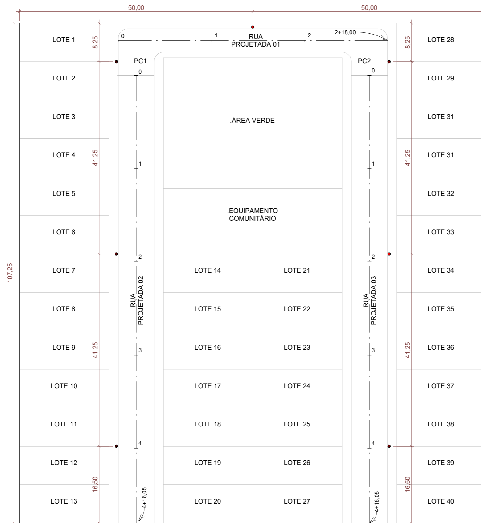
2 PLANTA BAIXA ESCALA 1 : 500
