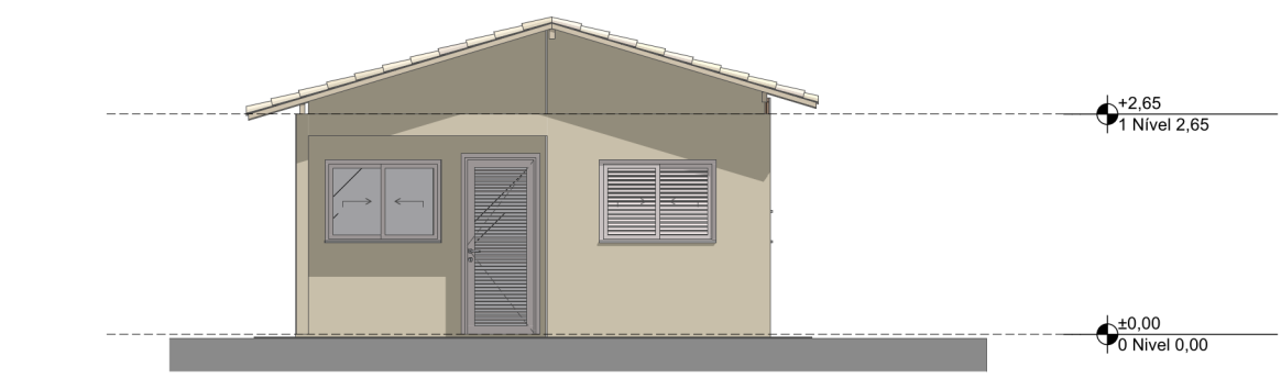
Elevação Frontal 1:100
