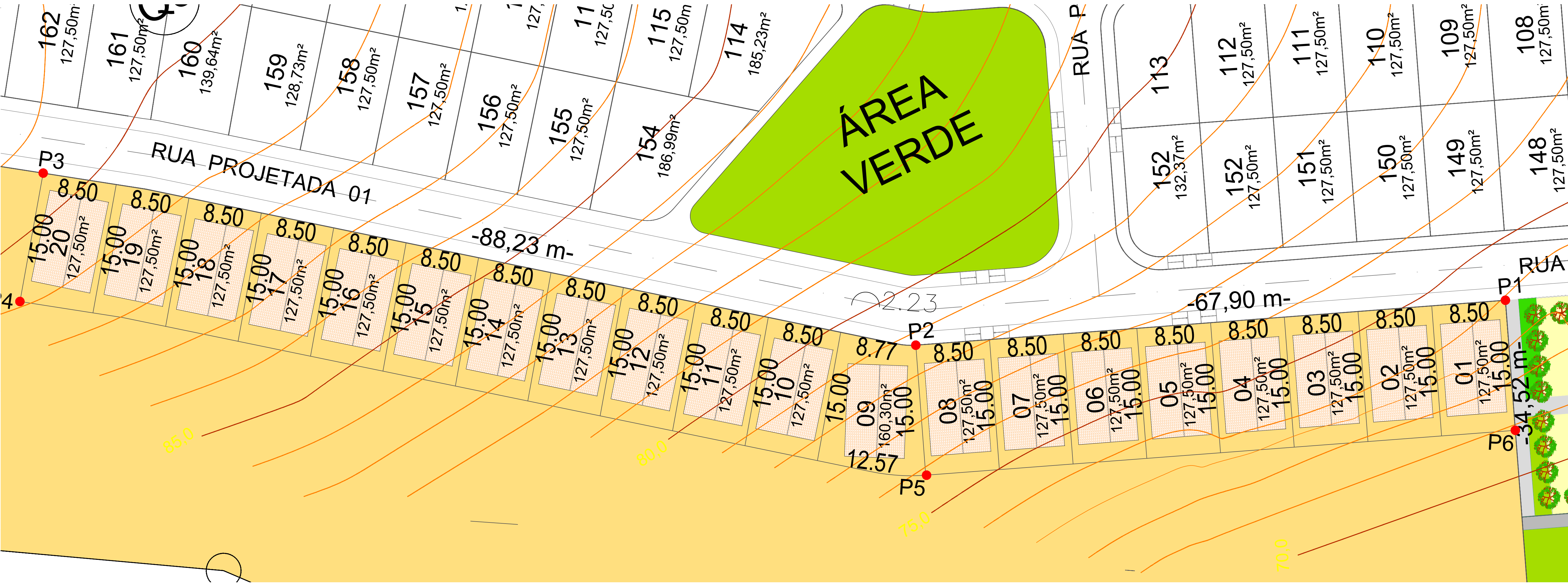
PLANTA DE LOCAÇÃO E COBERTA - FNHIS 20 UNIDADES - DISTRITO DE BATATEIRA Esc.: 1/250
