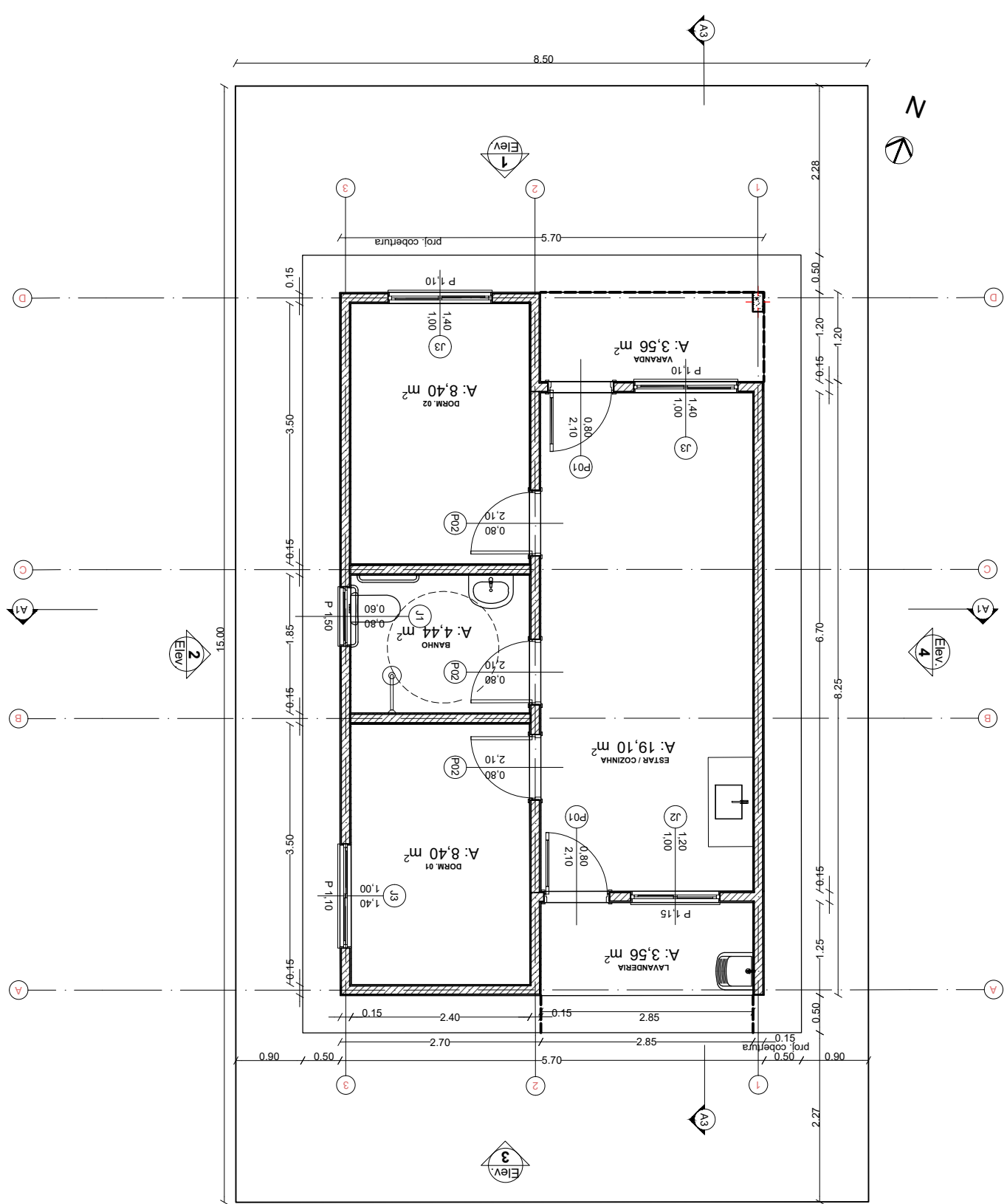
PLANTA DE IMPLANTAÇÃO Esc.: 1/75
