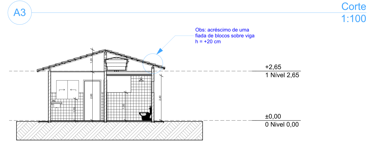
Corte 1:100
