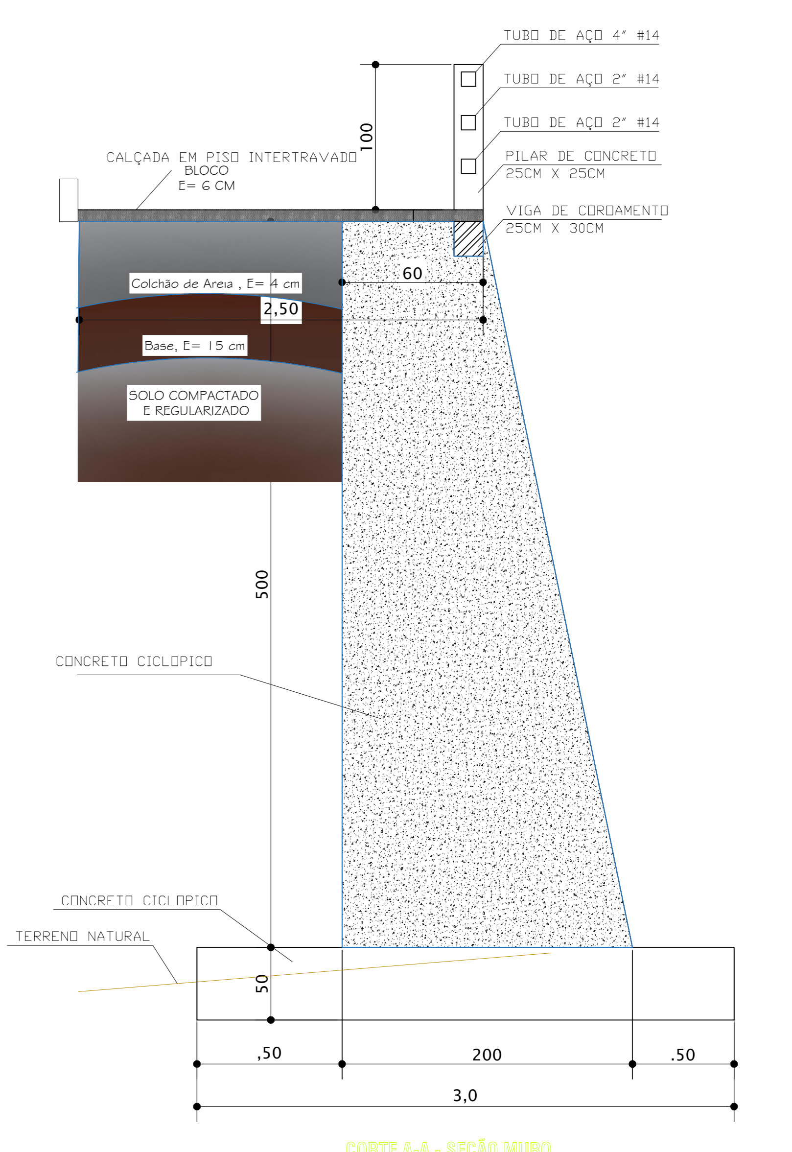
6 CORTE AA- SEÇÃO MURO ESCALA 1:200
