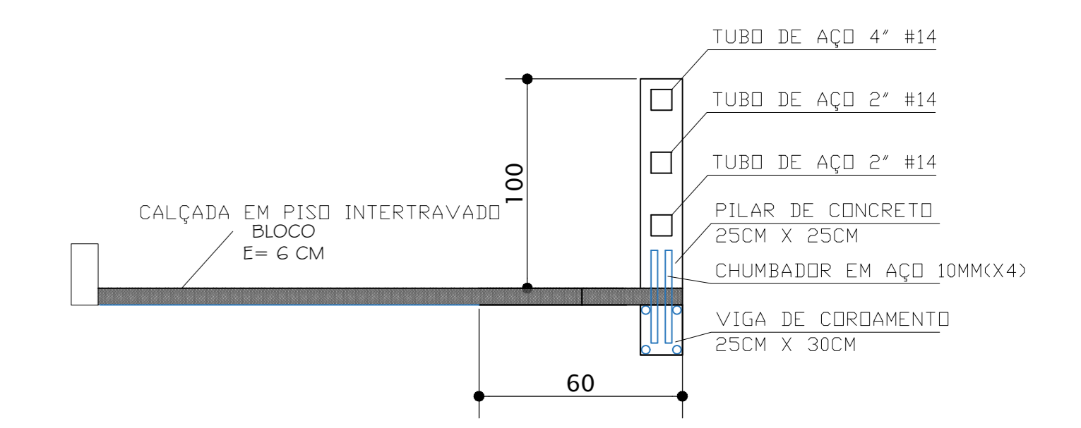
DET- 02
