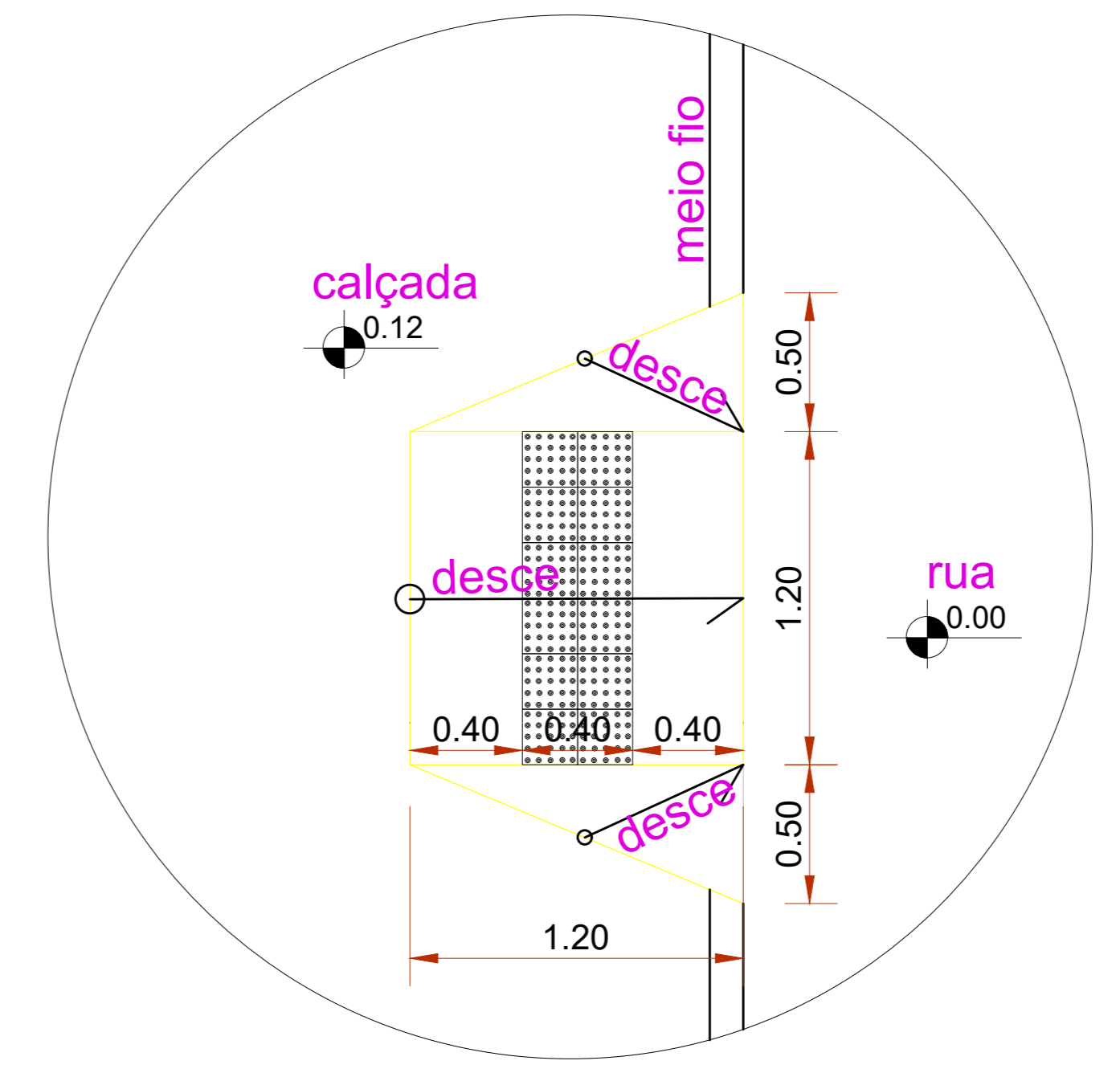
4 DETALHES ESCALA
