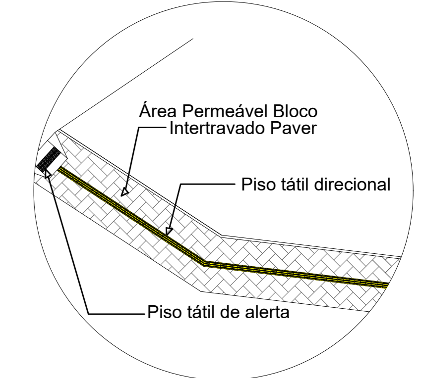
3 DETALHES ESCALA
