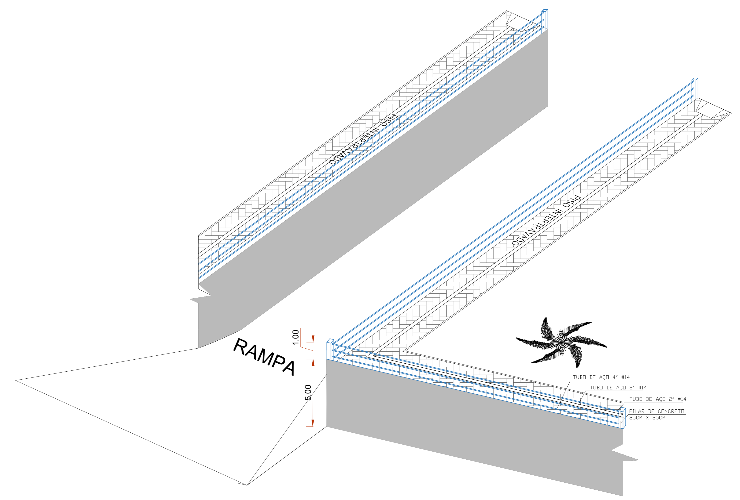
3 DETALHES ESCALA
