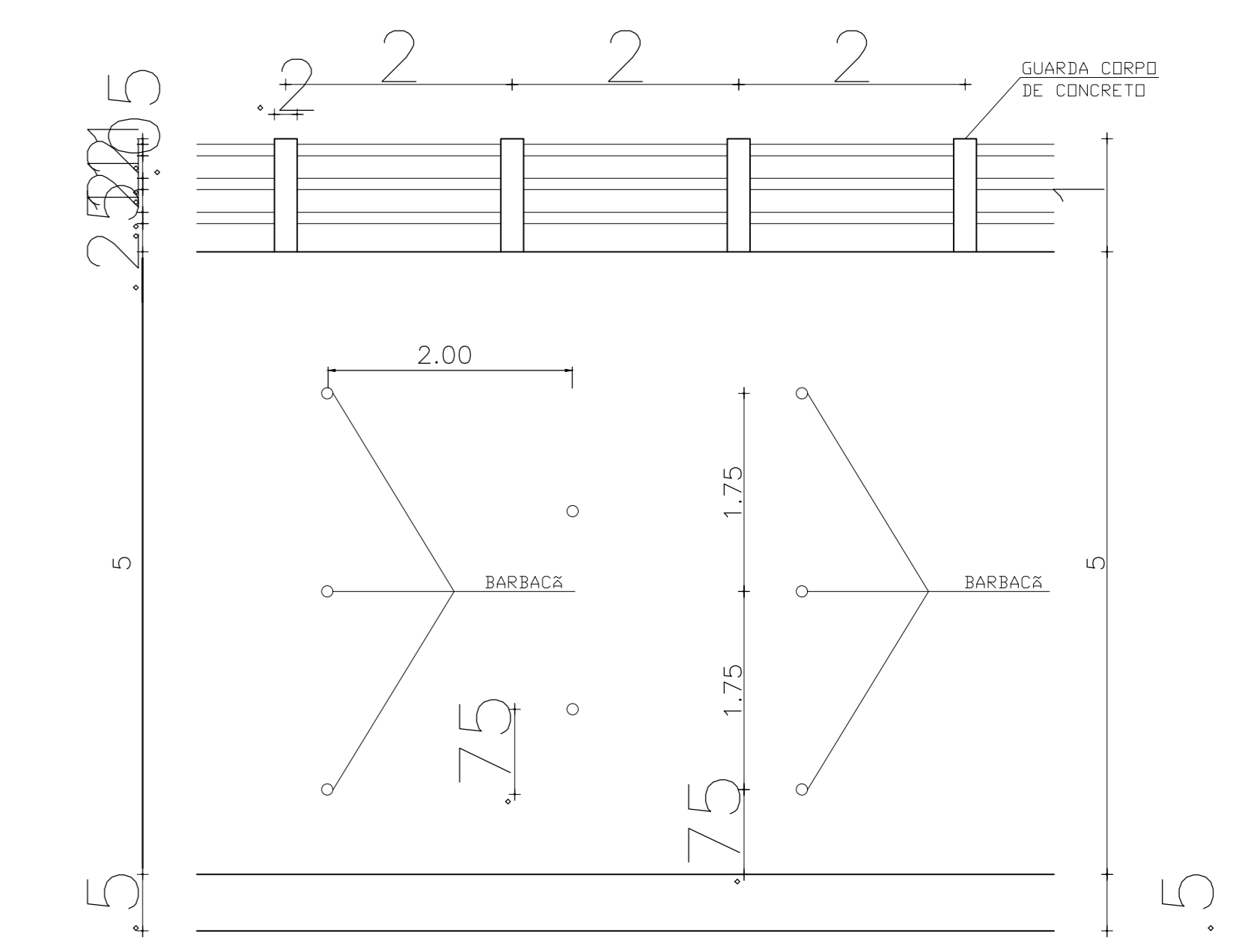
4 DETALHAMENTO FRONTAL MURO ESCALA 1:200
