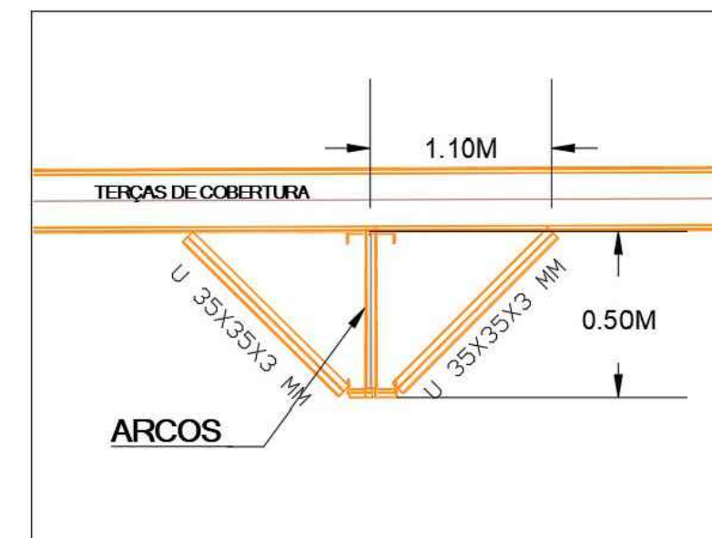
4 Detalhe- Mãos francesas SEM ESCALA
