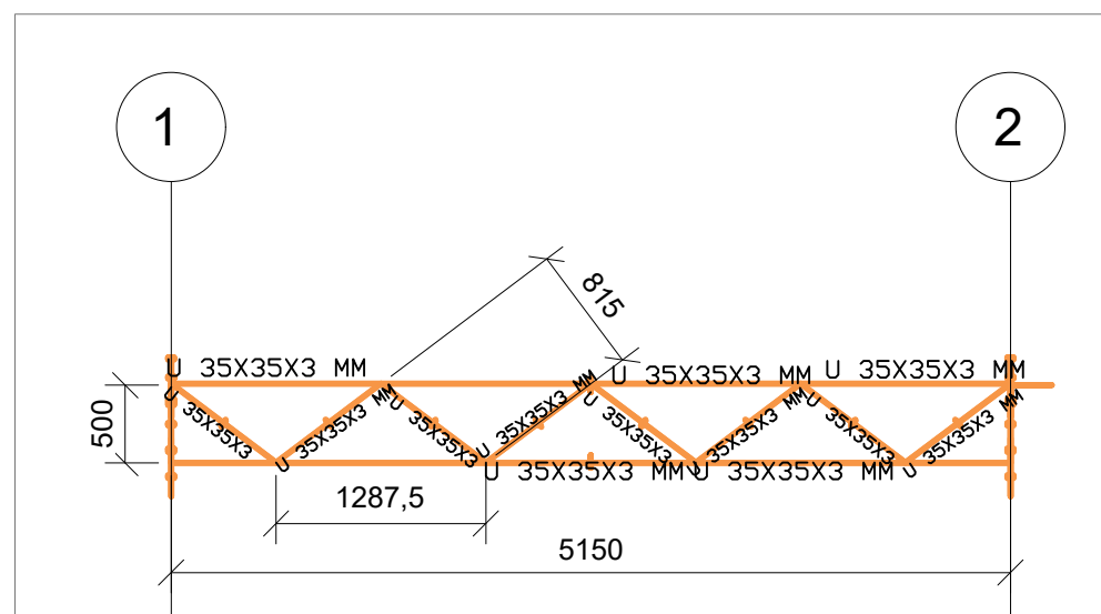
3 Detalhe- Vigas de rigidez(10 pçs) 1 : 50
