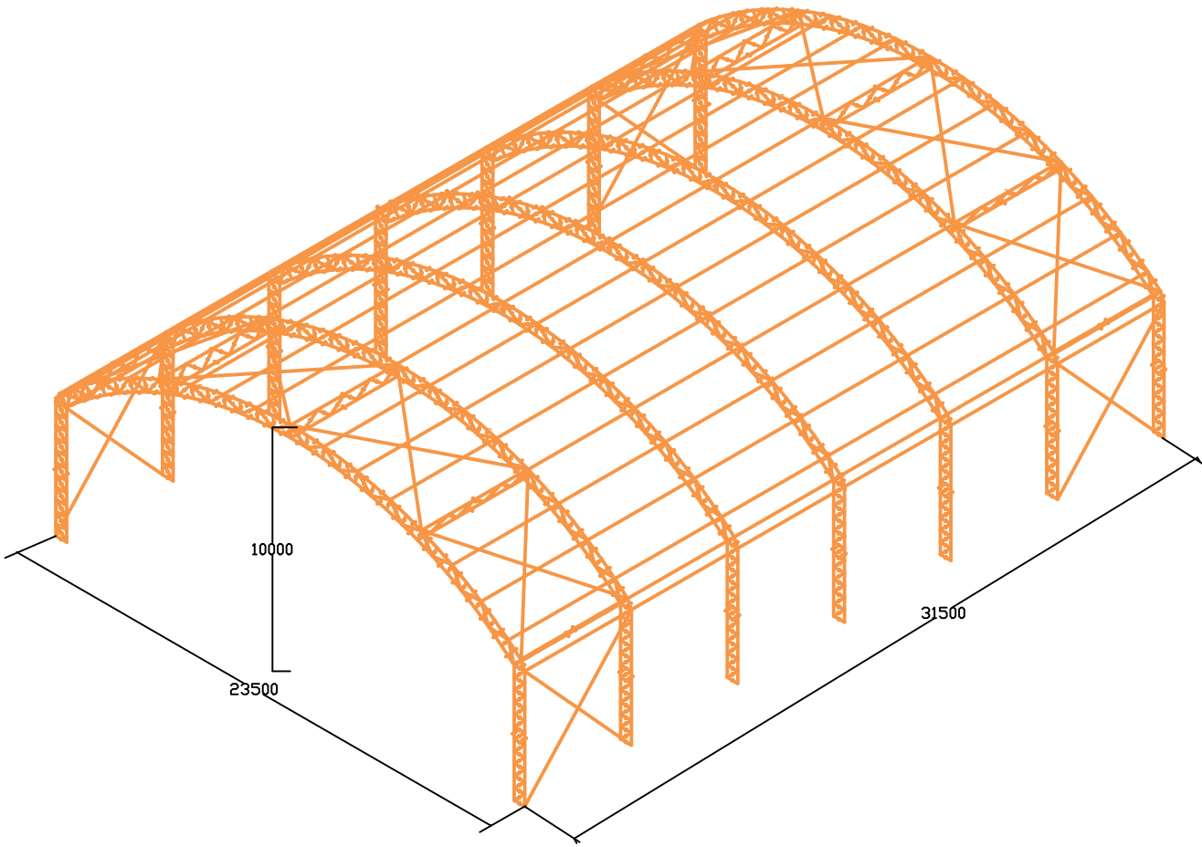
5 Vista isométrica ESCALA 1:300
