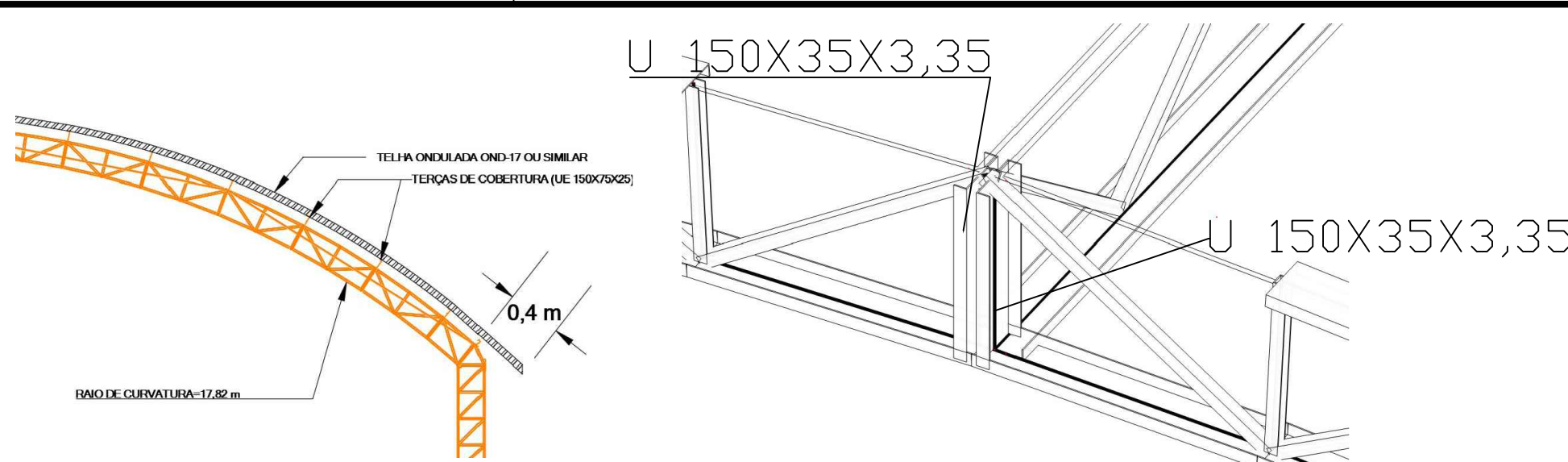
3 Detalhe da cobertura metálica SEM ESCALA
