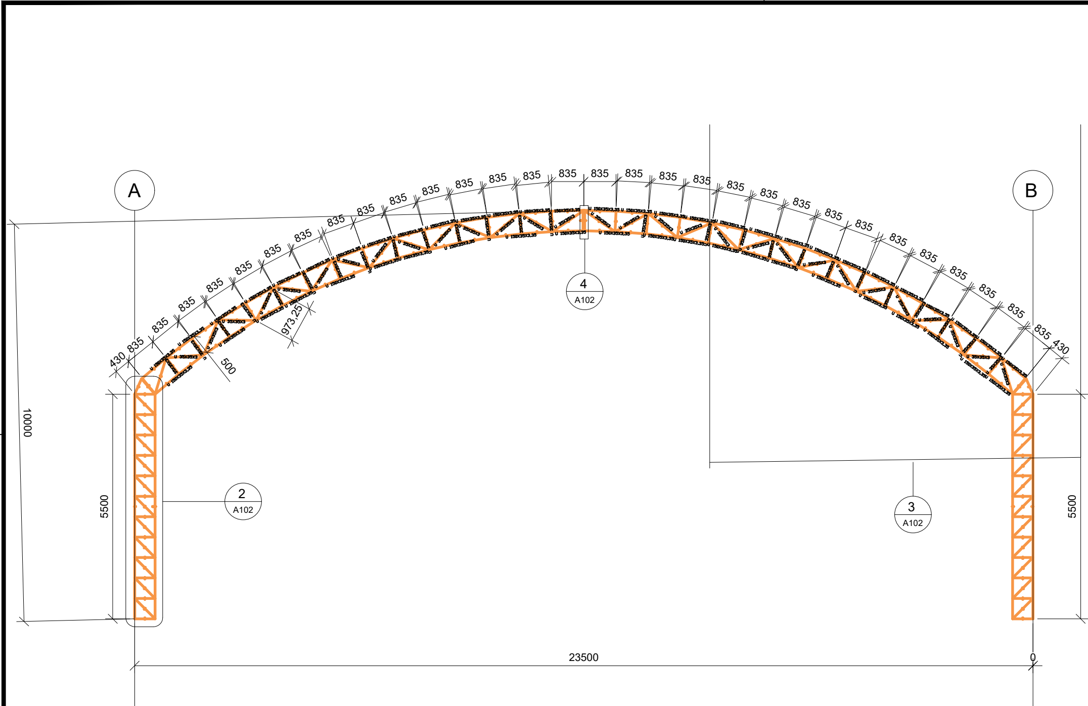
1 Vista frontal do arco ESCALA 1 : 100
