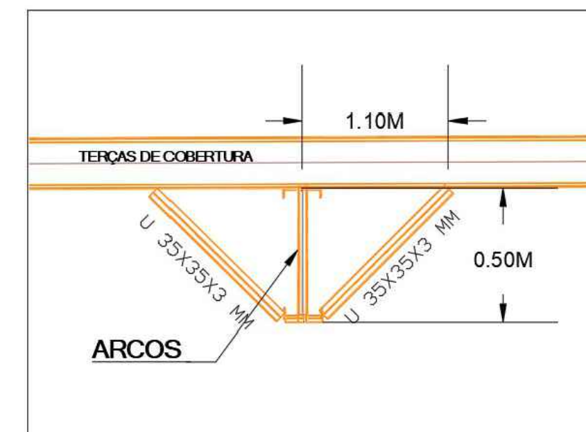
4 Detalhe- Mãos francesas SEM ESCALA
