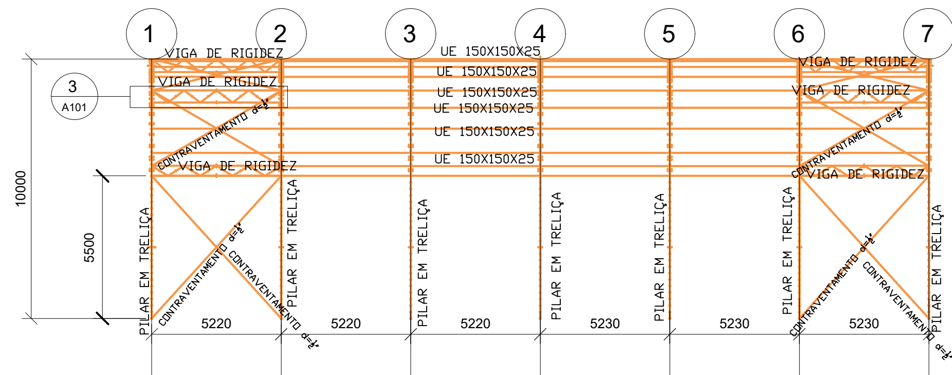
1 Detalhe- Vista Lateral Esquerda 1 : 150
