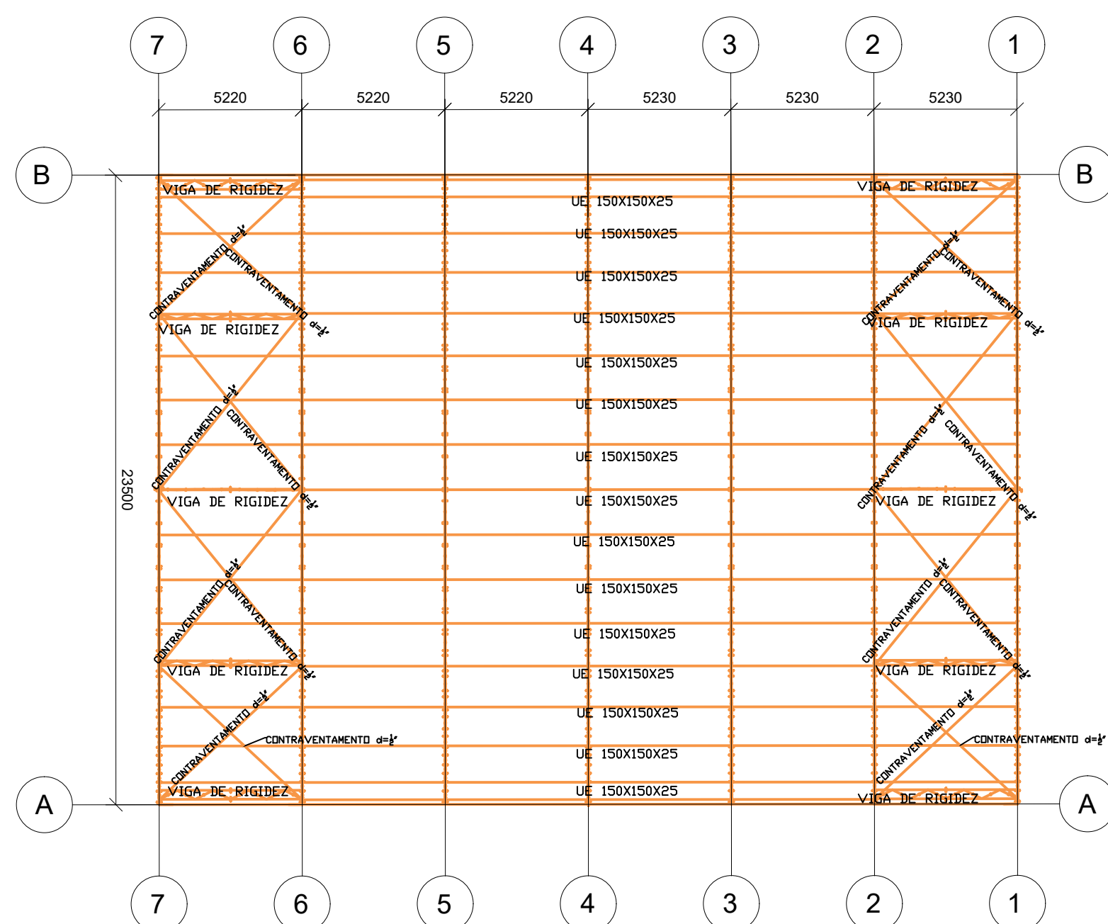
2 Detalhe- Vista Superior 1 : 200
