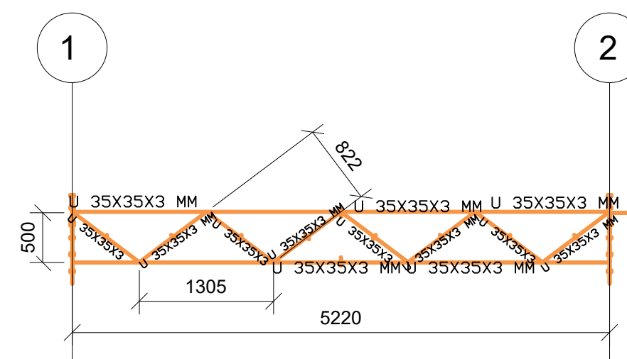
3 Detalhe- Vigas de rigidez(10 pçs) 1 : 50
