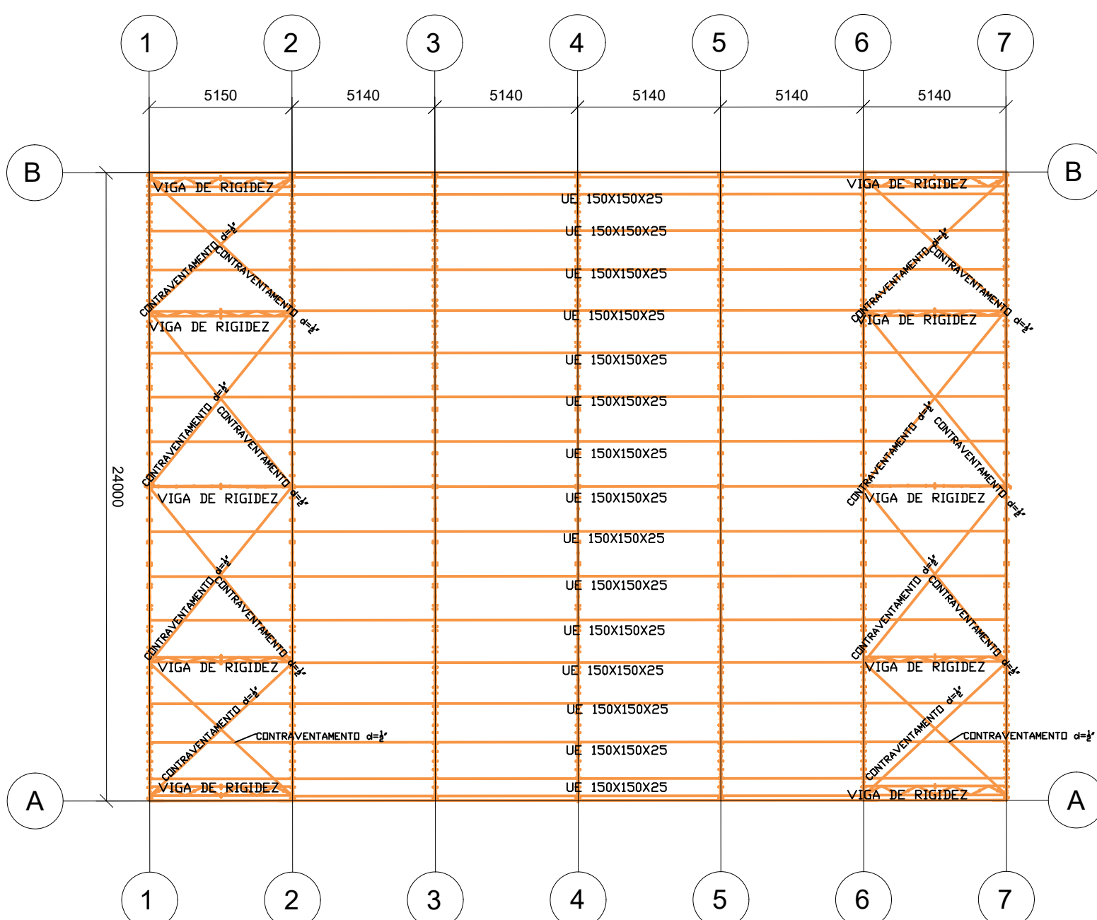
2 Detalhe- Vista Superior 1 : 200
