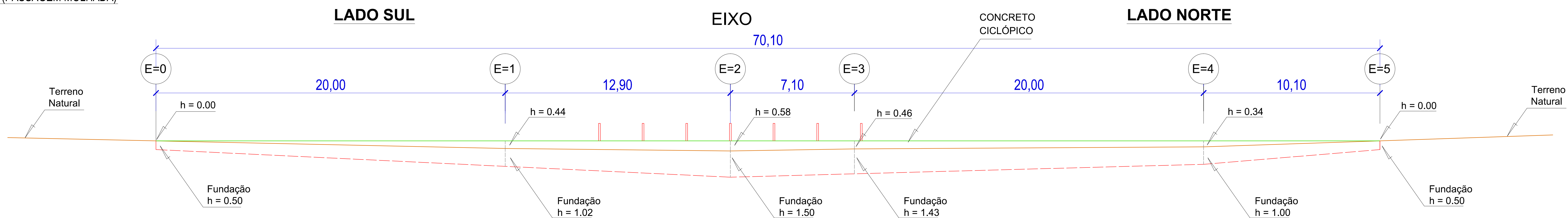
2 VISTA LONGITUDINAL (PASSAGEM MOLHADA) Esc. 1/100
