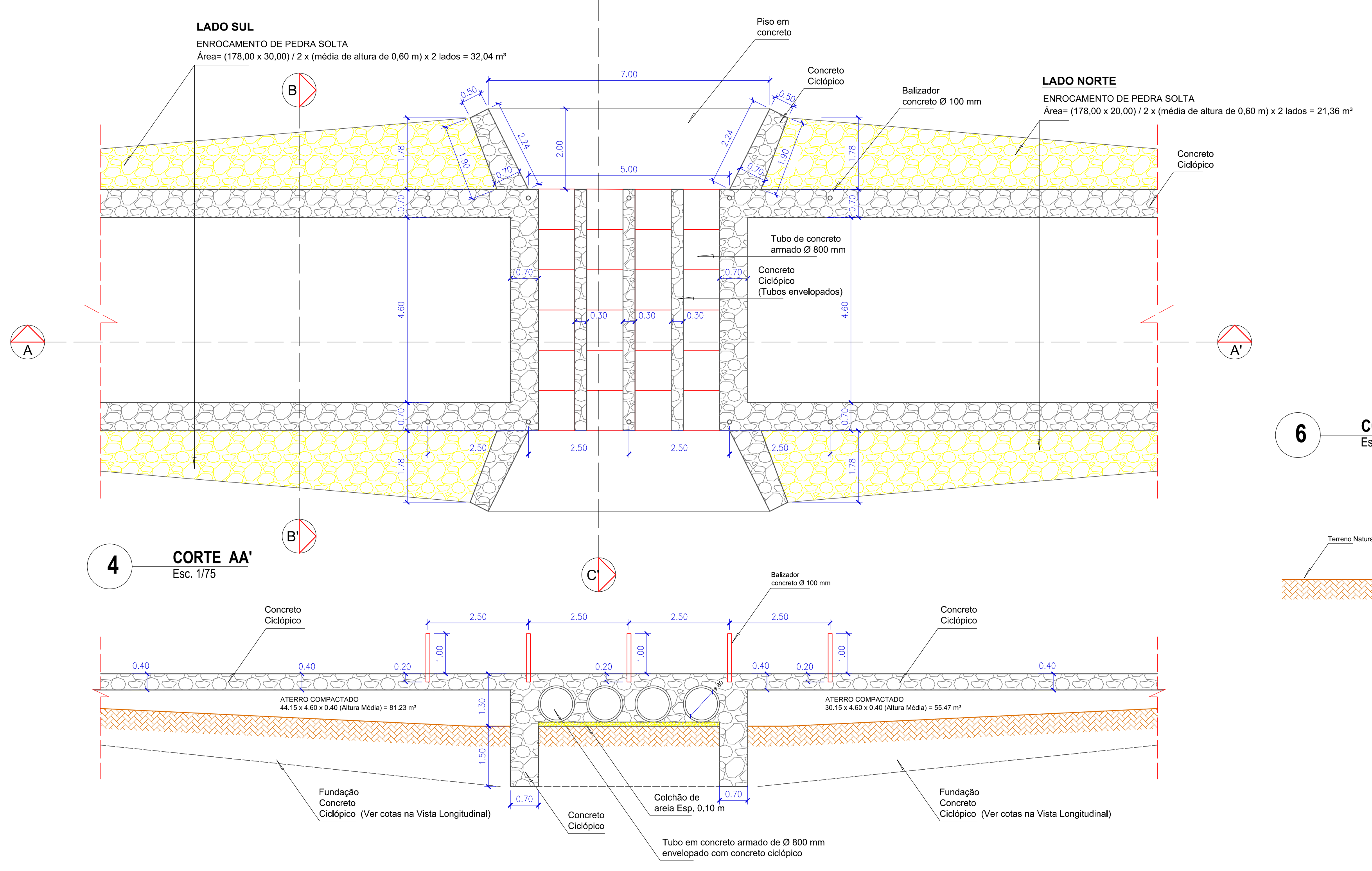
3 PLANTA BAIXA (BUEIRO) Esc. 1/75
