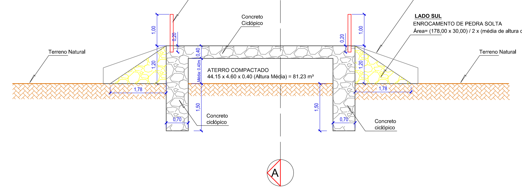
6 CORTE BB' Esc. 1/75
