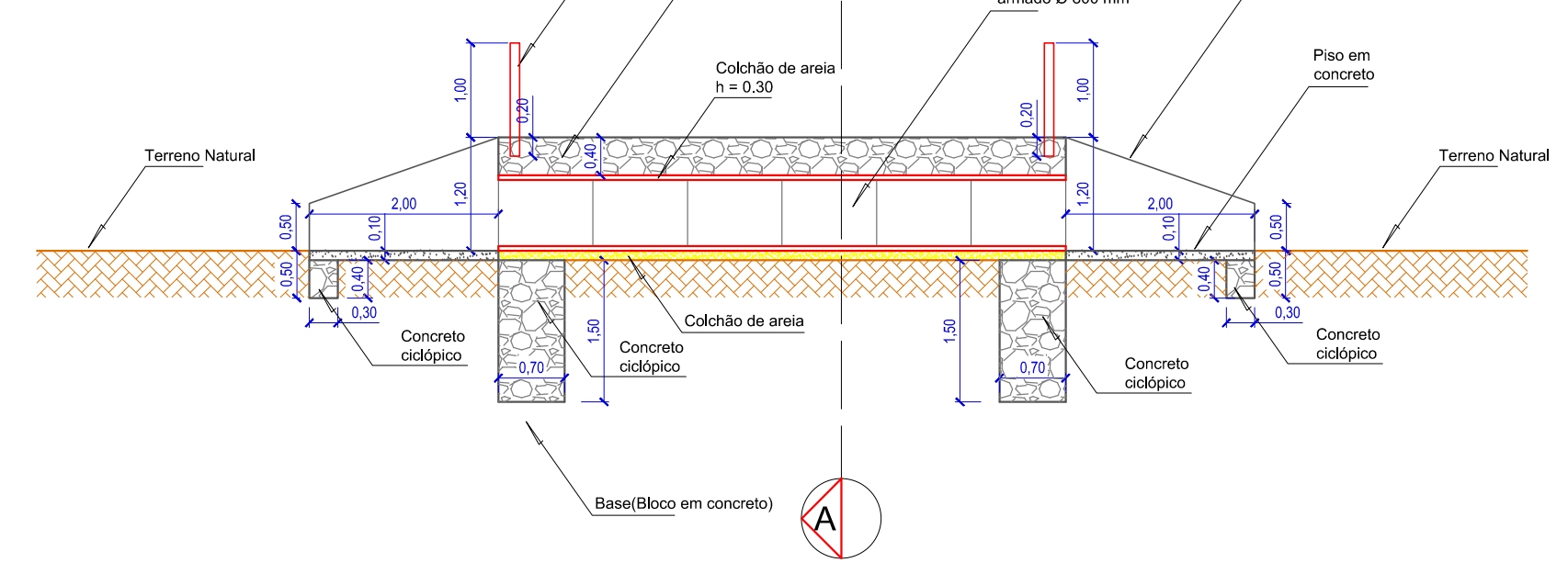
7 CORTE CC' Esc. 1/75
