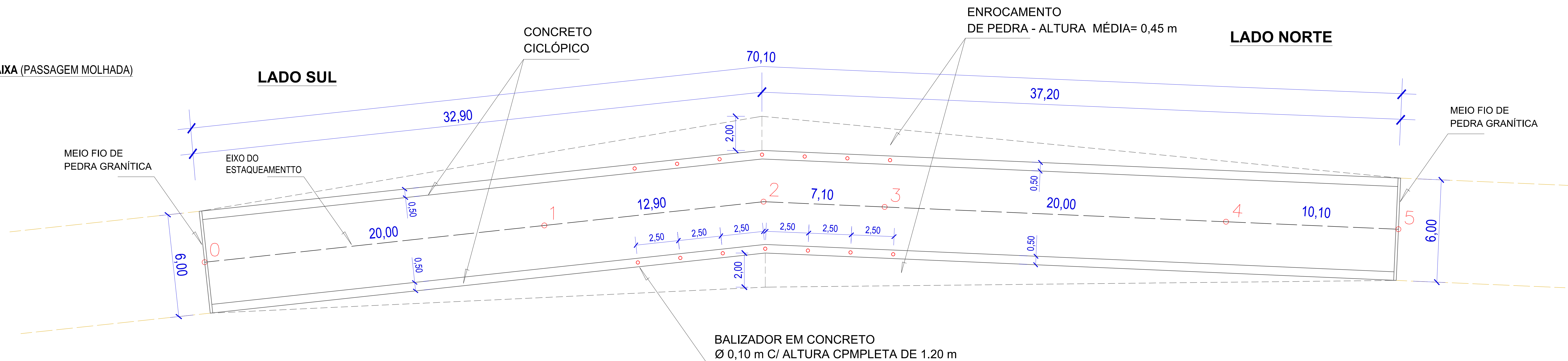
2 VISTA LONGITUDINAL (PASSAGEM MOLHADA) Esc. 1/100
