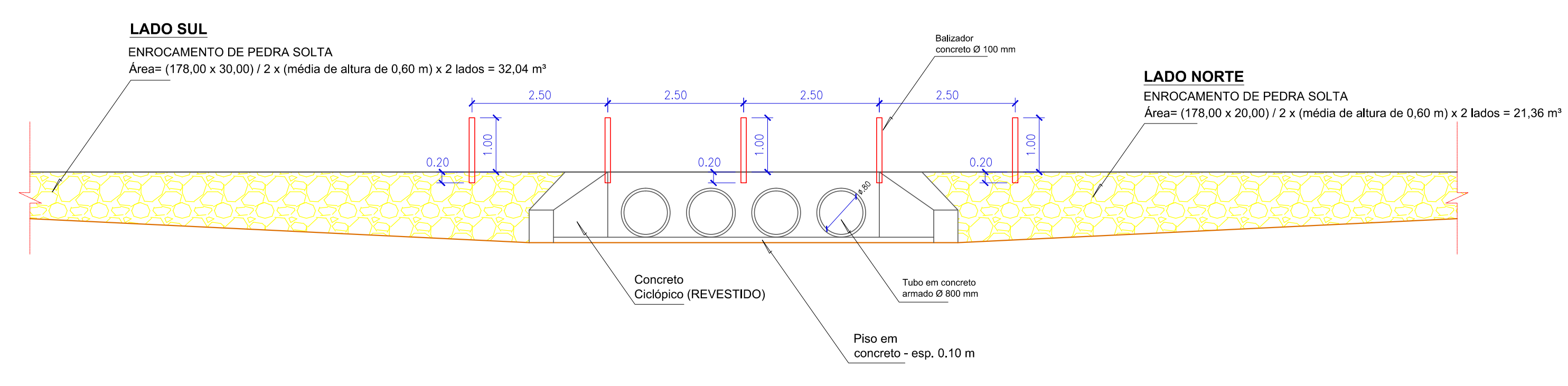
5 VISTA LATERAL Esc. 1/75
