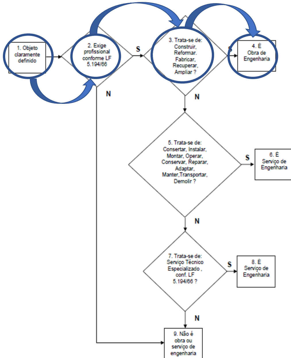
Figura 2 - Fluxograma para enquadramento do tipo de obra (IBRAOP OT- IBR 002/2009)
