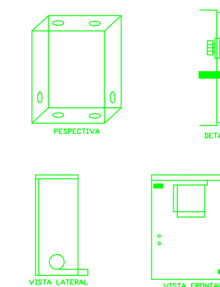
CAIXA METÁLICA PARA MEDIDOR DE ENERGIA
