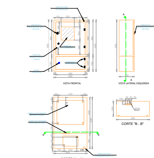
CORTE B-B
