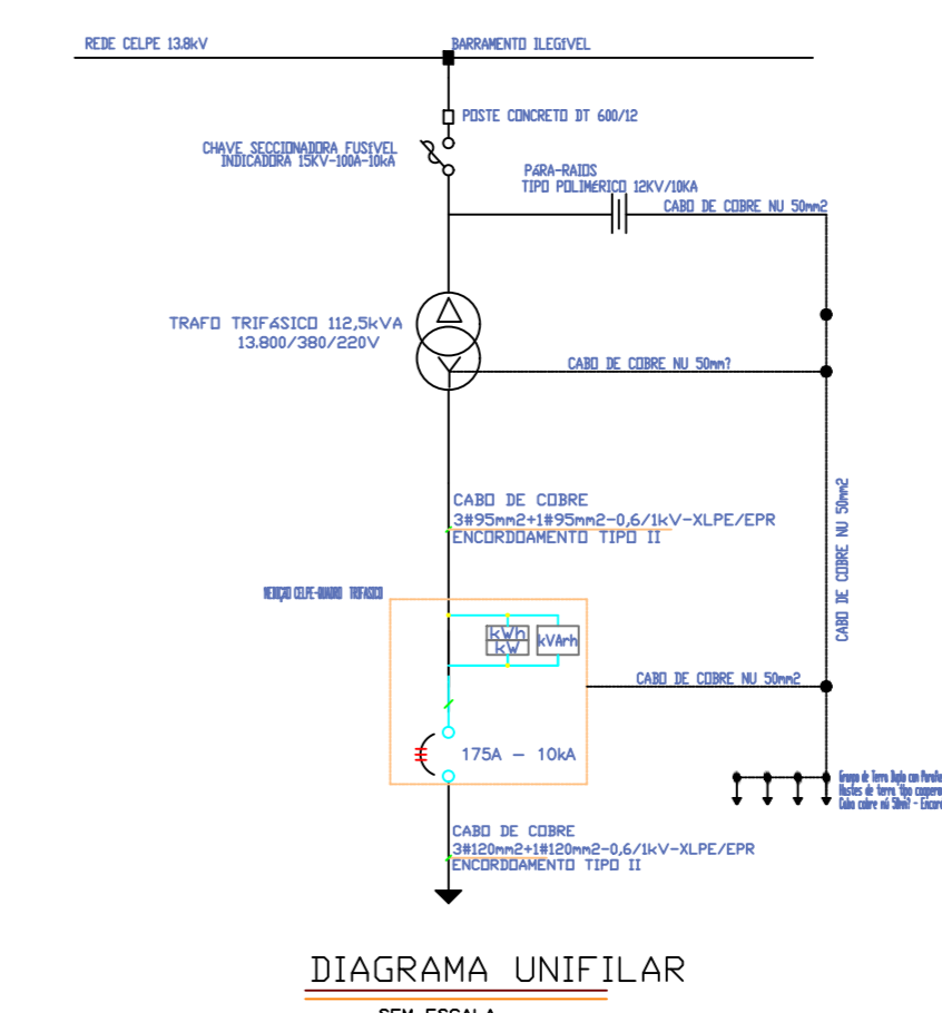
DIAGRAMA UNIFILAR SEM ESCALA
