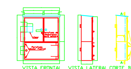
CAIXA METÁLICA F3
