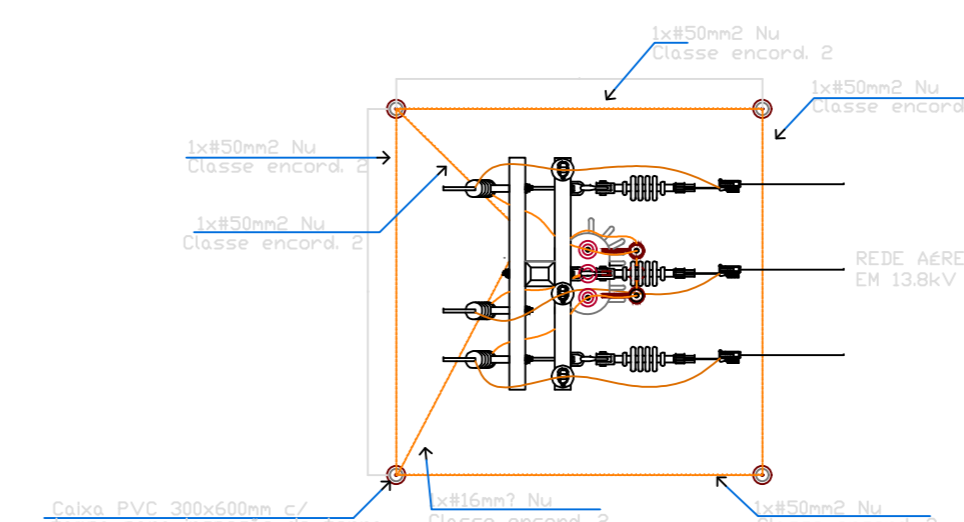
VISTA SUPERIOR ESCALA 1:50
