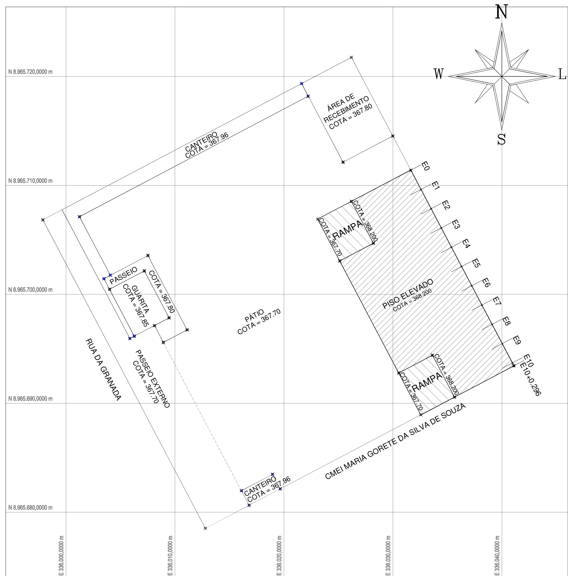
LEV. PLANIALT. - ECOPONTO (Parte 02) Esc.: 1/200
