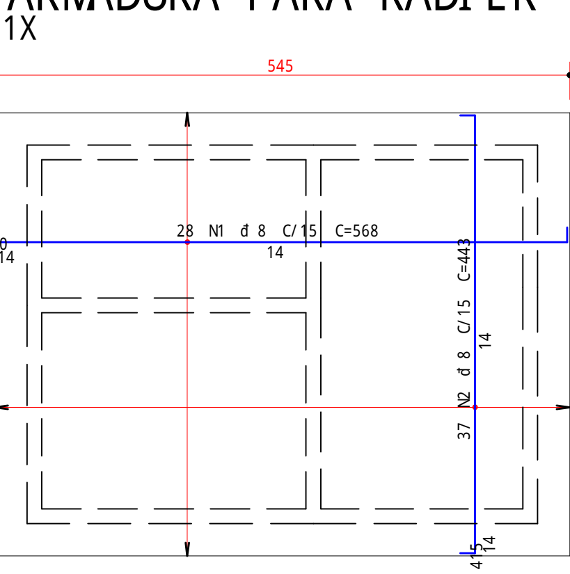
ARM . POS. RADIER H=16cm ESC. 1/50
