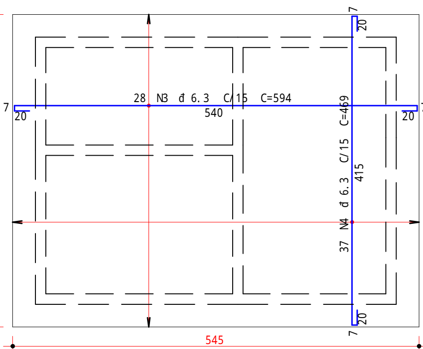
ARM . NEG. LAJ E H=10cm ESC. 1/50
