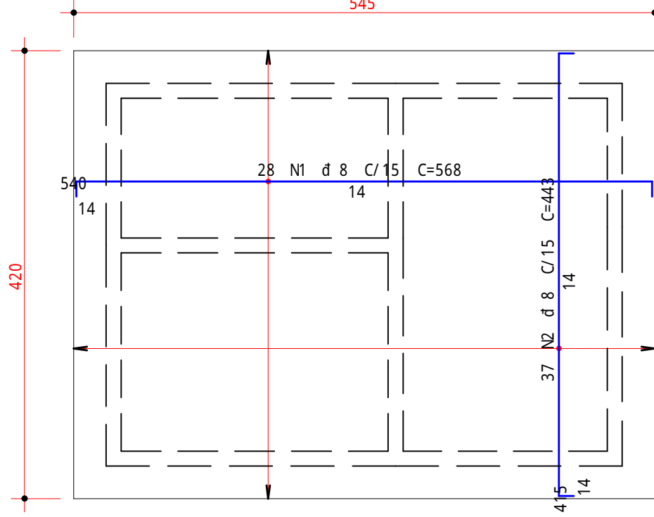
ARM . NEG. RADIER H=16cm ESC. 1/50
