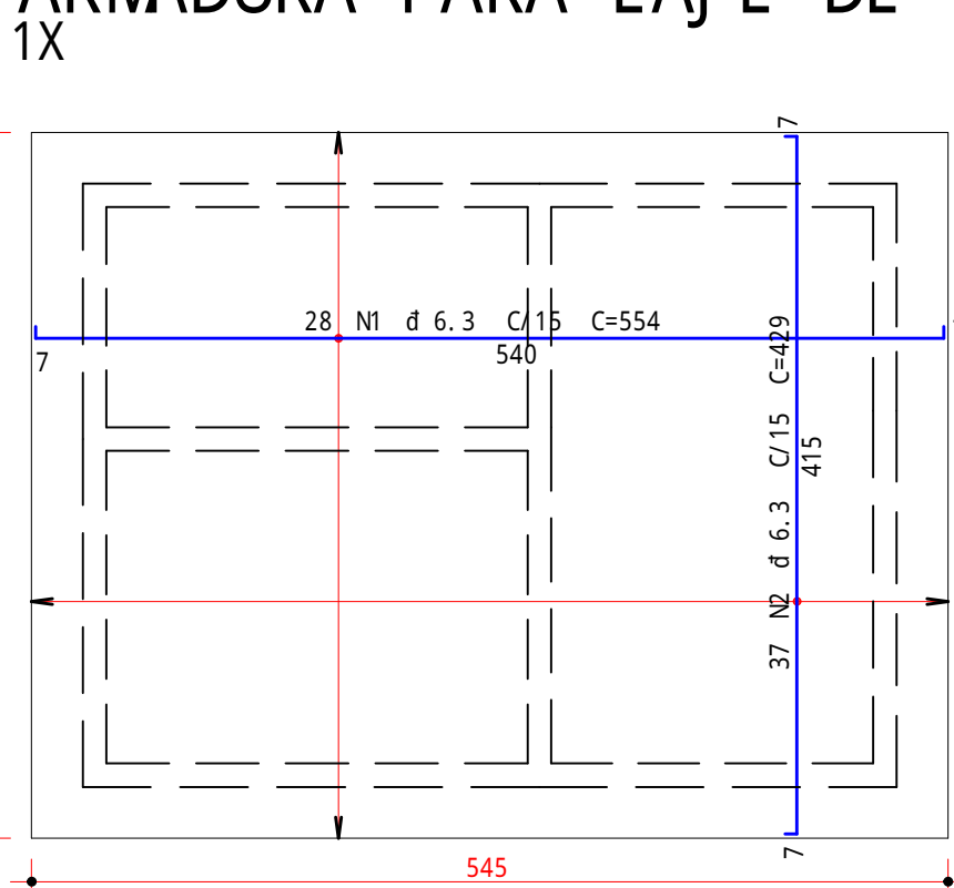
ARM . POS. LAJ E H=10cm ESC. 1/50
