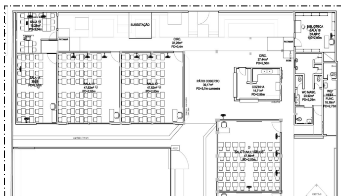
Figura 22 – Planta Baixa Layout – Trecho 2 - Escola Parque – Bloco 3. Fonte: Gerência de Engenharia, 2024.
