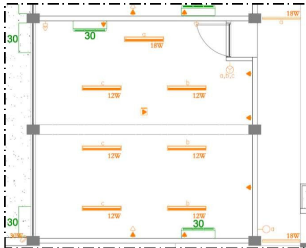
Figura 26 – Distribuição das seções e pontos de luz em sala de aula tipo.
