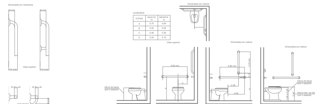
DETALHES BARRAS DE APOIO
