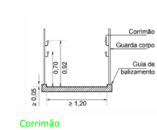
Corrimão
