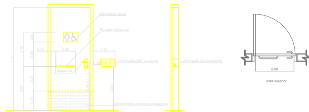
DETALHE SINALIZAÇÃO DE PORTAS
