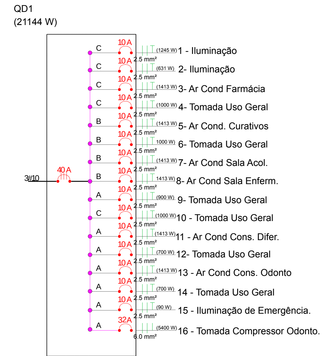
Diagrama Unifilar esc.: 1:50
