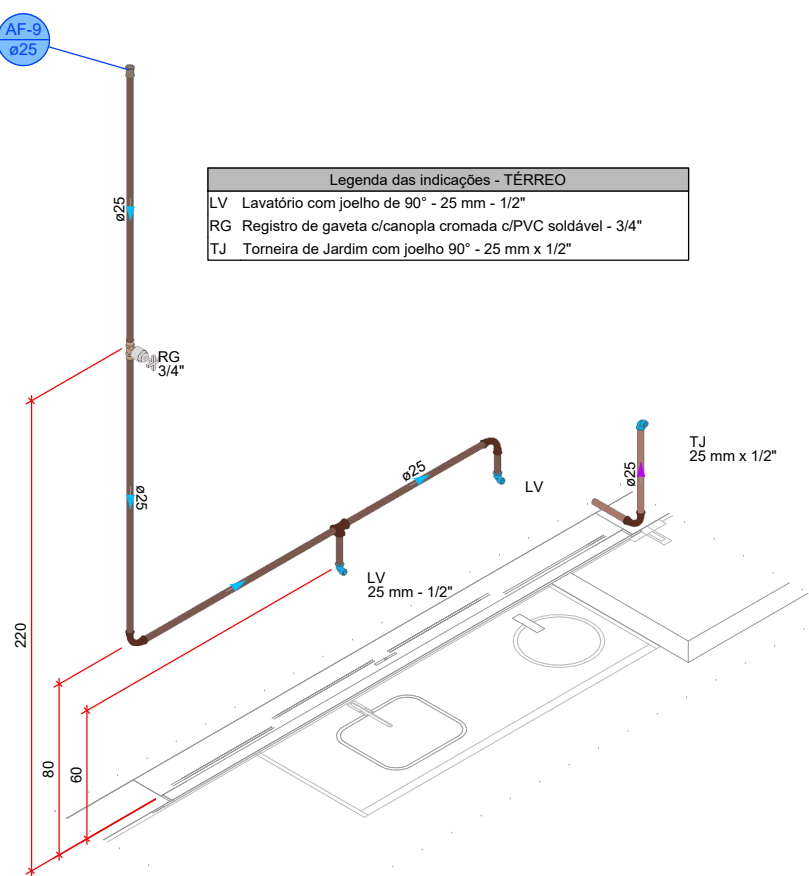
DETALHE HID-11 1:25
