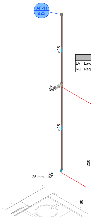
DETALHE HID-9 1:25
