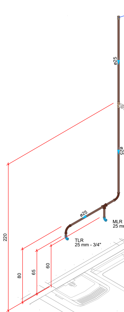
DETALHE HID-6 1:25
