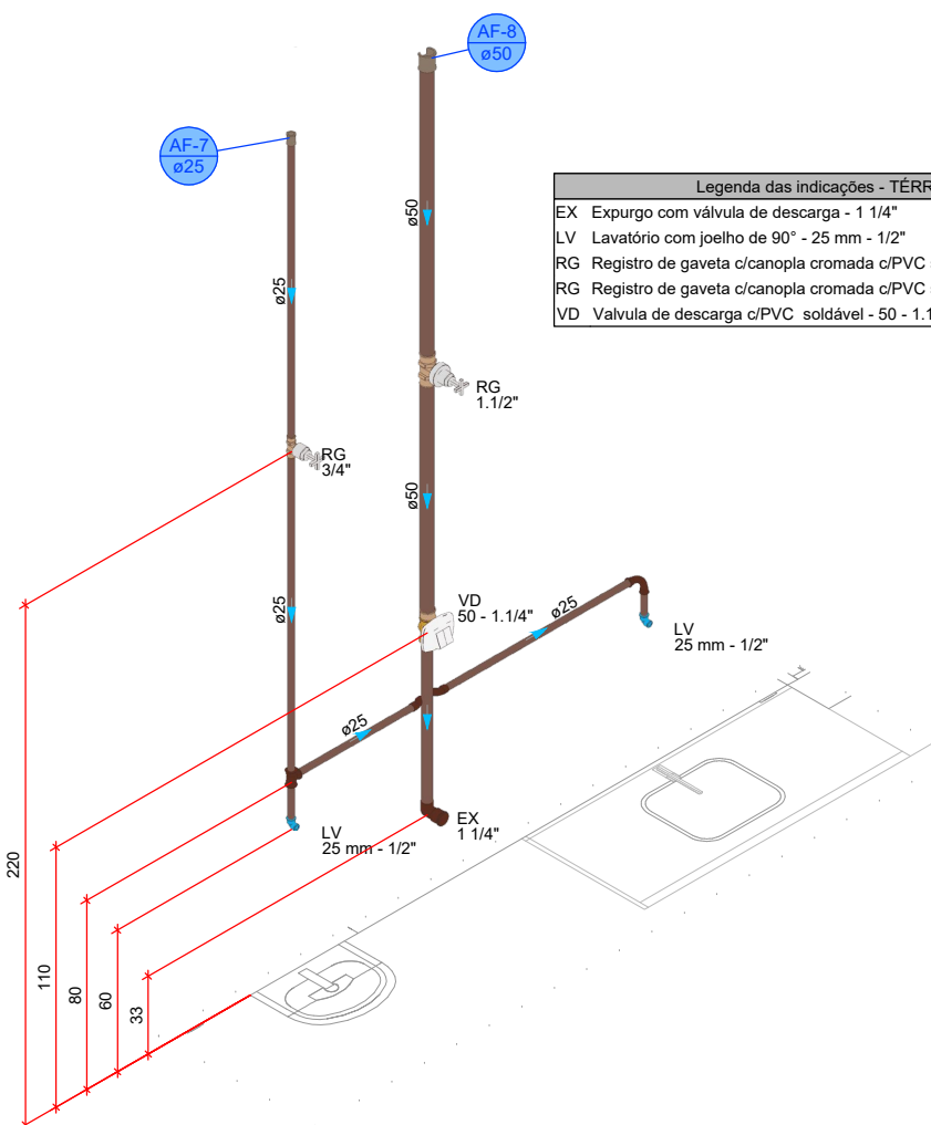
DETALHE HID-8 1:25
