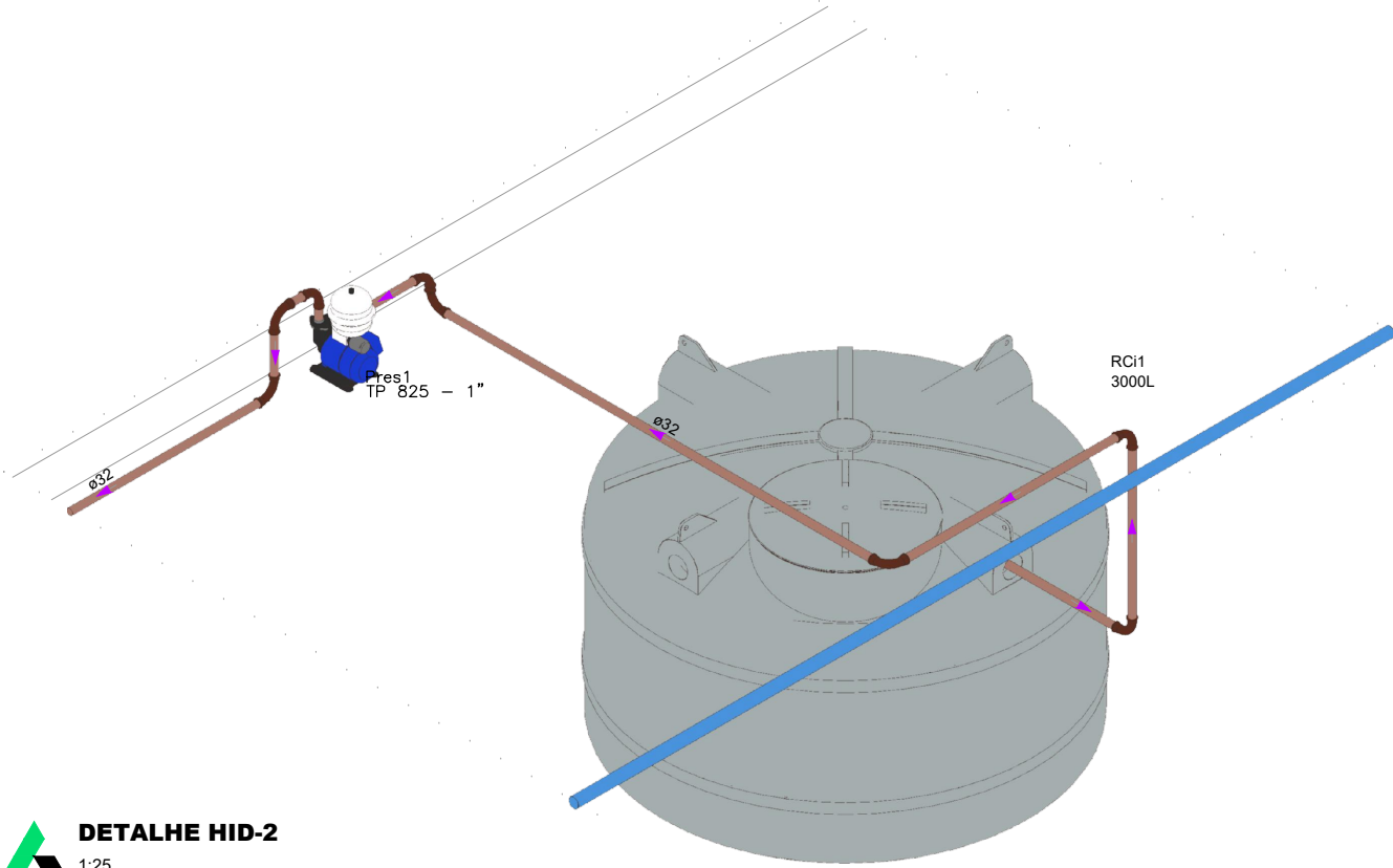
DETALHE HID-2 1:25
