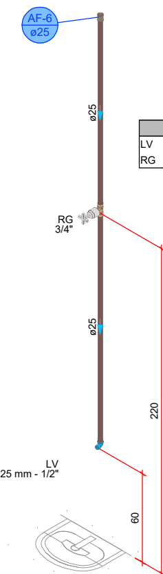
DETALHE HID-7 1:25
