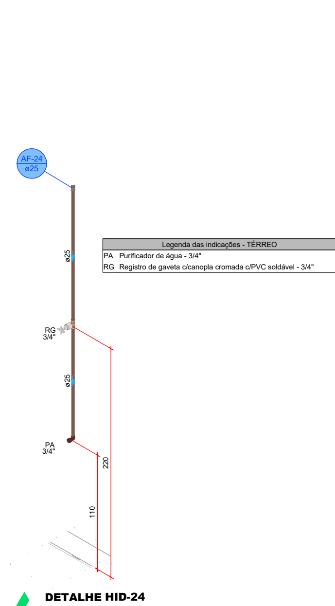
DETALHE HID-24 1:25
