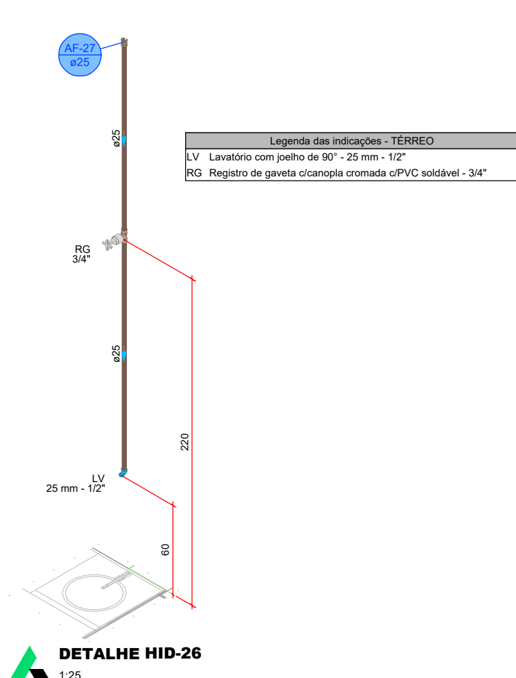
DETALHE HID-26 1:25
