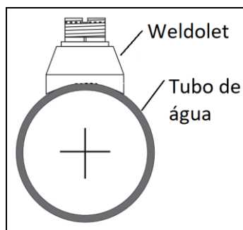
Figura 1: Desenho esquemático do Weldolet instalado.
