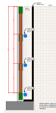
3 DRENAGEM 1:25
