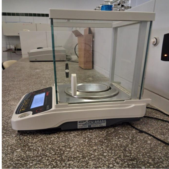
Figura 40 – Vista lateral balança 04.
