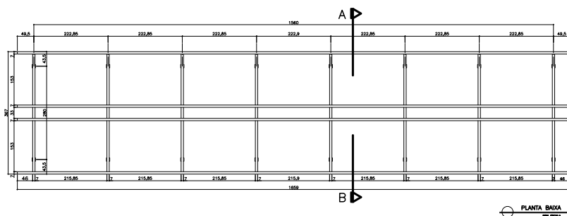
PAINEL FOTOVOLTÁICO 16 ESTACAS
