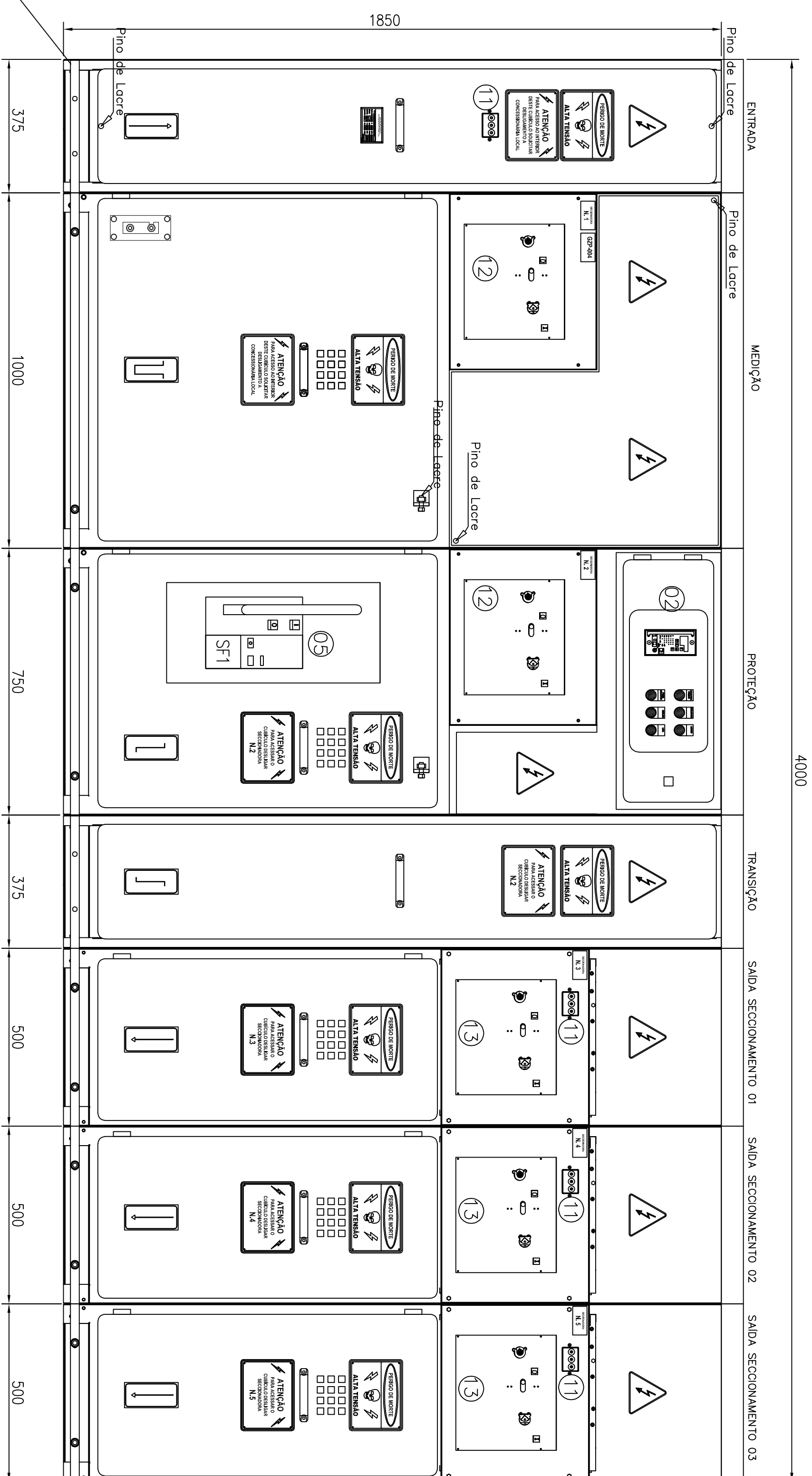
VISTA FRONTAL ESCALA 1:20
