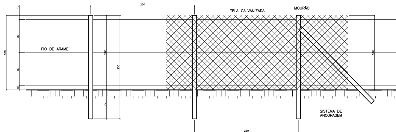
CERCA ALAMBRADO SEM ESCALA
