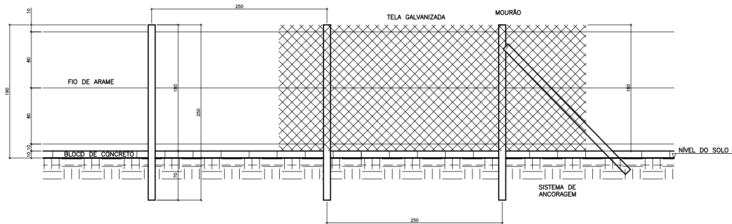
CERCA ALAMBRADO COM BASE DE BLOCO SEM ESCALA
