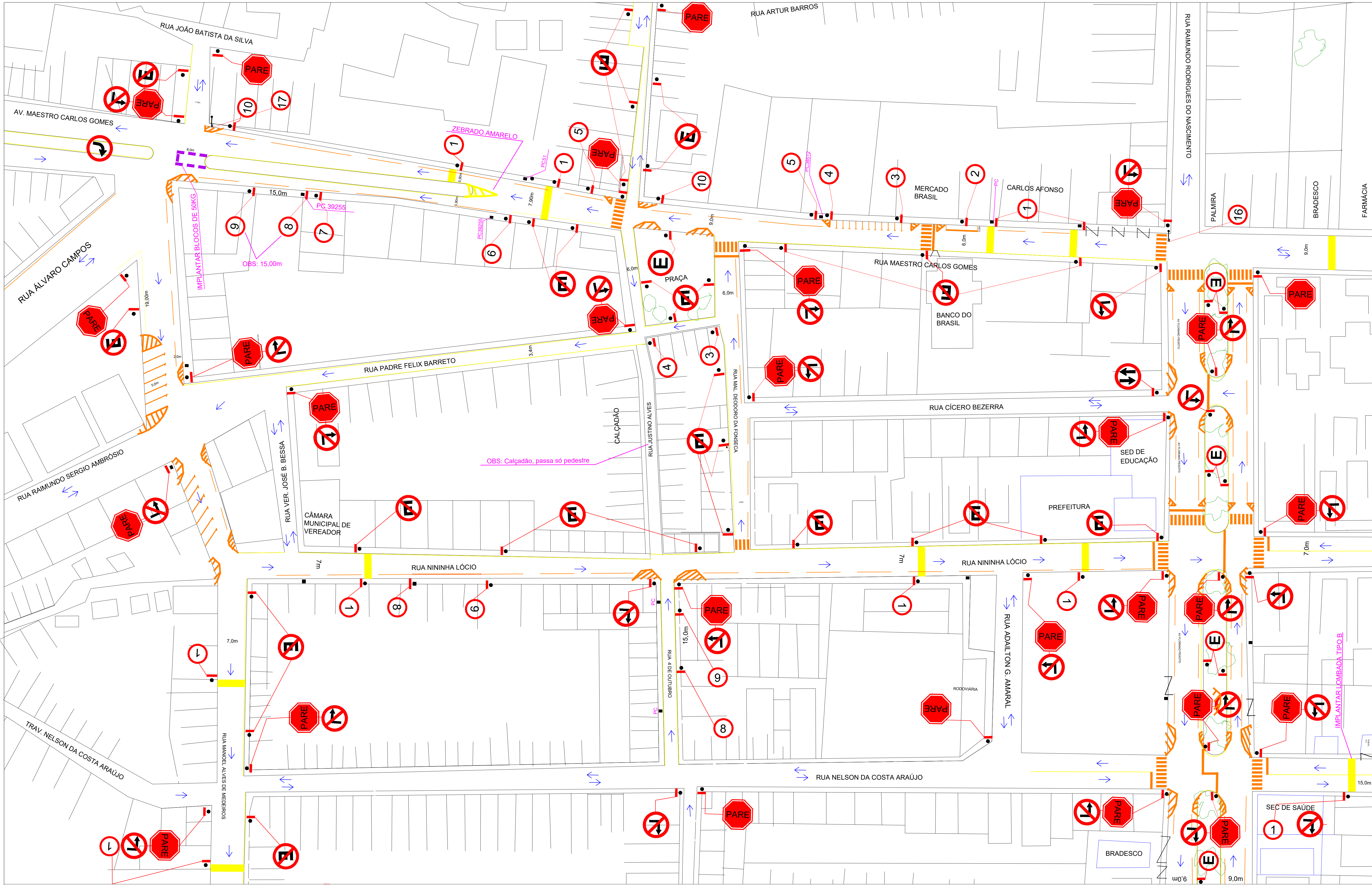
2 Planta de Sinalização - Trecho 01 Sem Escala
